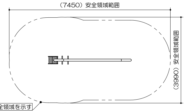
安全領域範囲 S= 1 : 100
