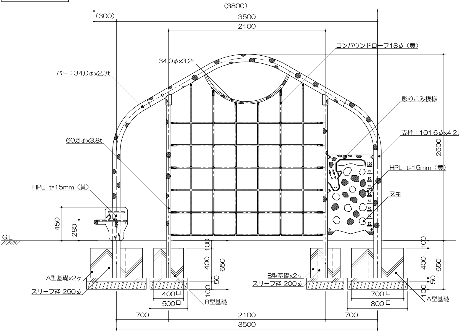
立面図 S= 1 : 30
