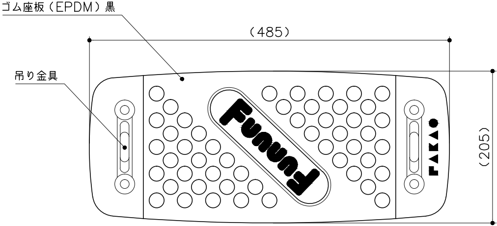
平面図 S=1:5
