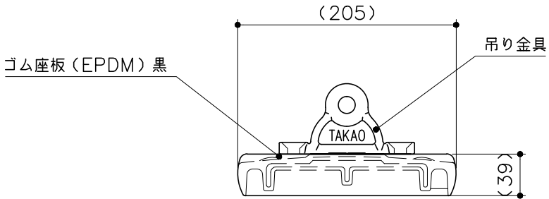
側面図 S=1:5
