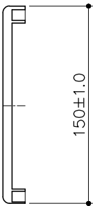
A-A'断面
