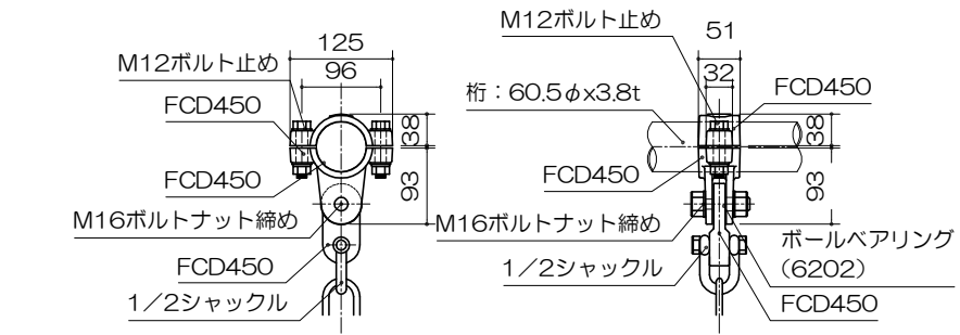
H=2500 (中央部) 継手詳細図 S= 1 : 10
