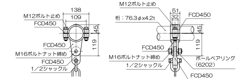
H=2500部 ブランコハンガー詳細図 S= 1 : 10
