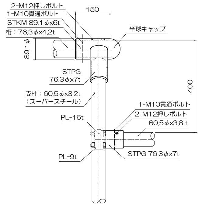
H=2500 (中央部) 継手詳細図 S= 1 : 10
