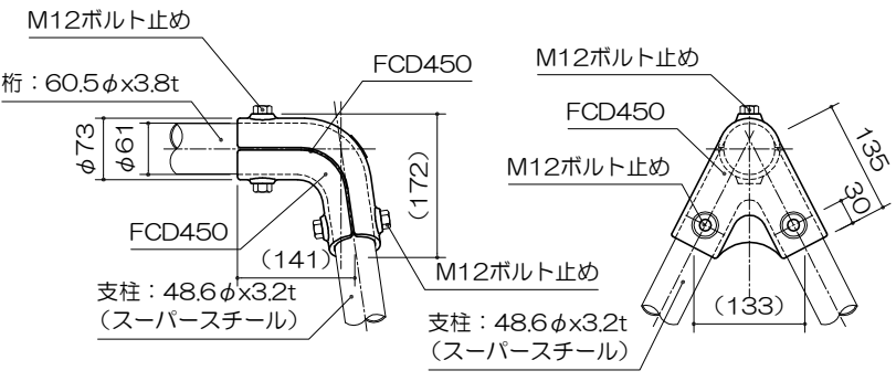
H=2100部 角イモノ詳細図 S= 1 : 10
