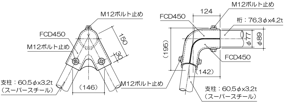
H=2500部 角イモノ詳細図 S= 1 : 10
