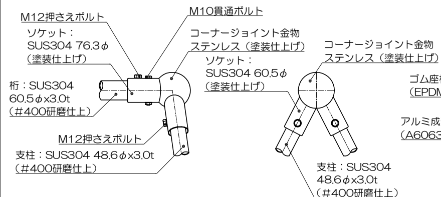
ブランコハンガー詳細図 S= 1 : 10
