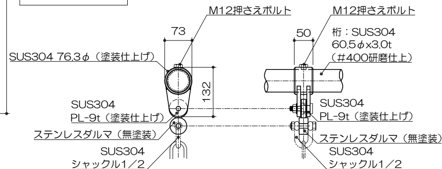
側面図 S= 1 : 60
