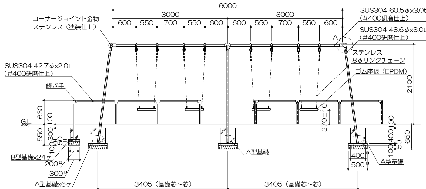
立面図 S= 1 : 60
