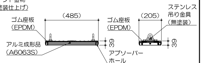
ゴム座板断面図 S= 1 : 20
