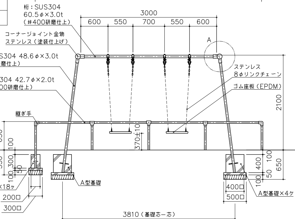
S= 1 : 50
