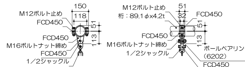
側面図
