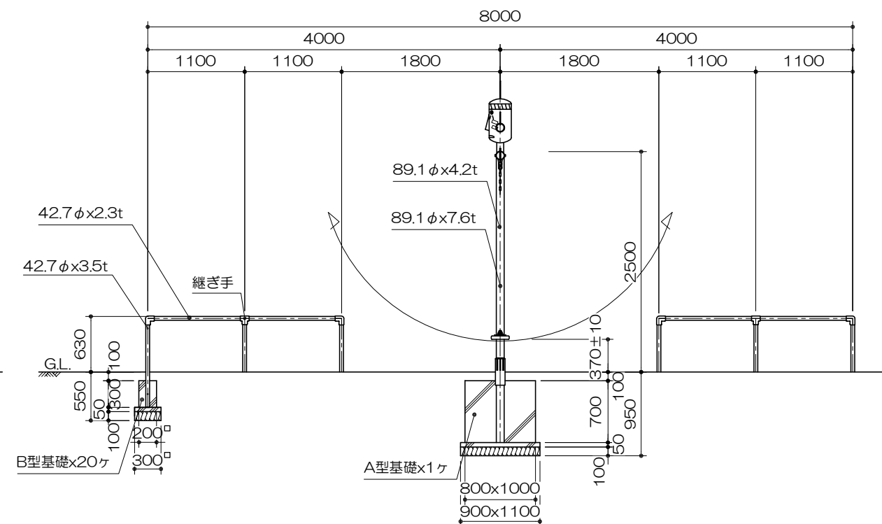
側面図
