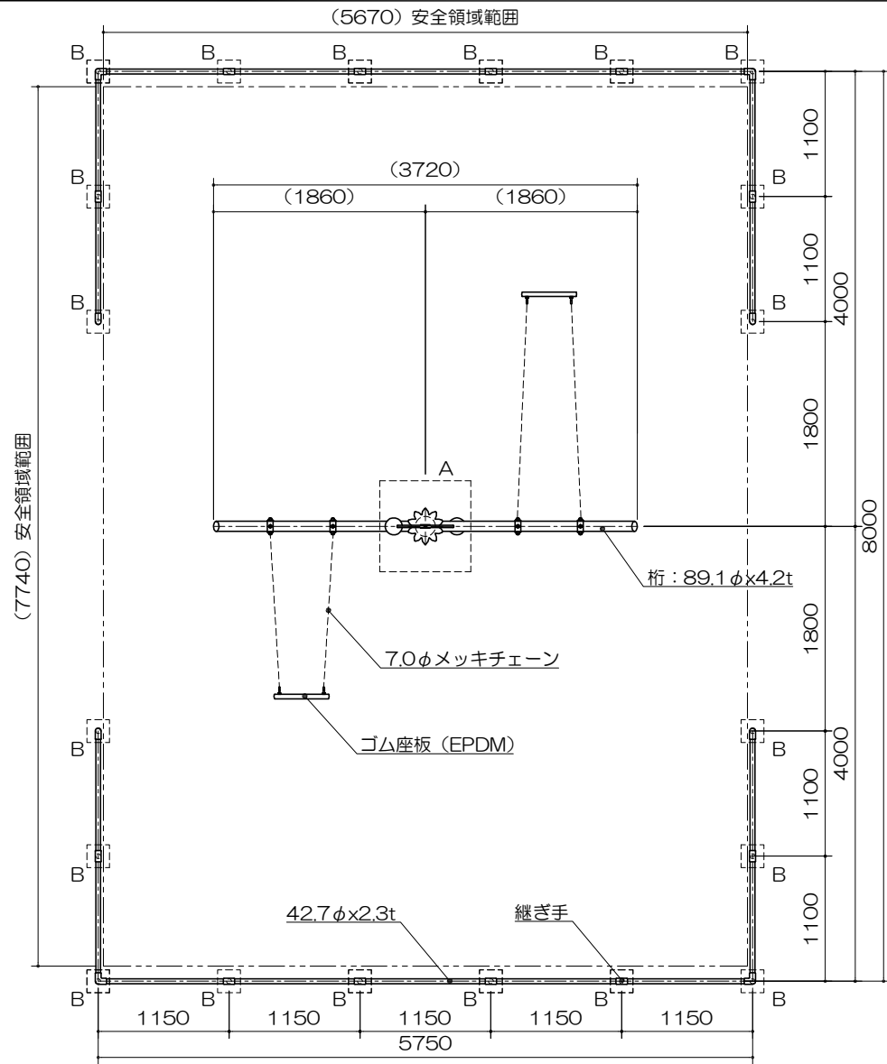
平面図 S= 1 : 60
