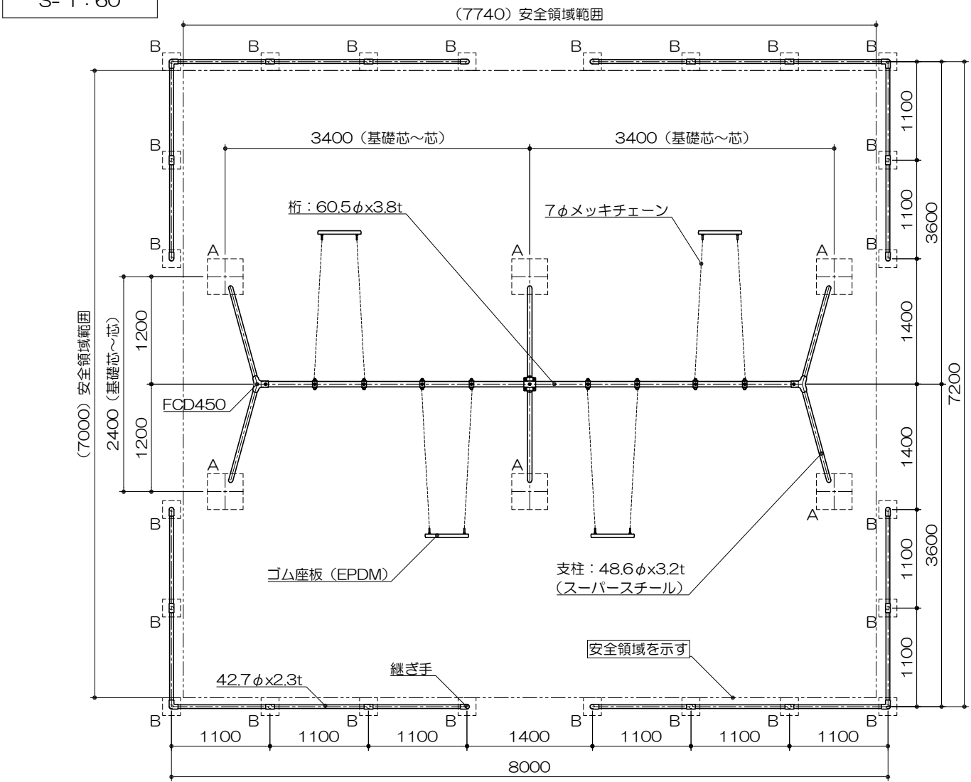
平面図 S= 1 : 60
