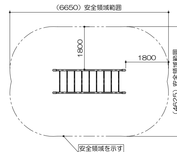
安全領域範囲 S= 1 : 100
