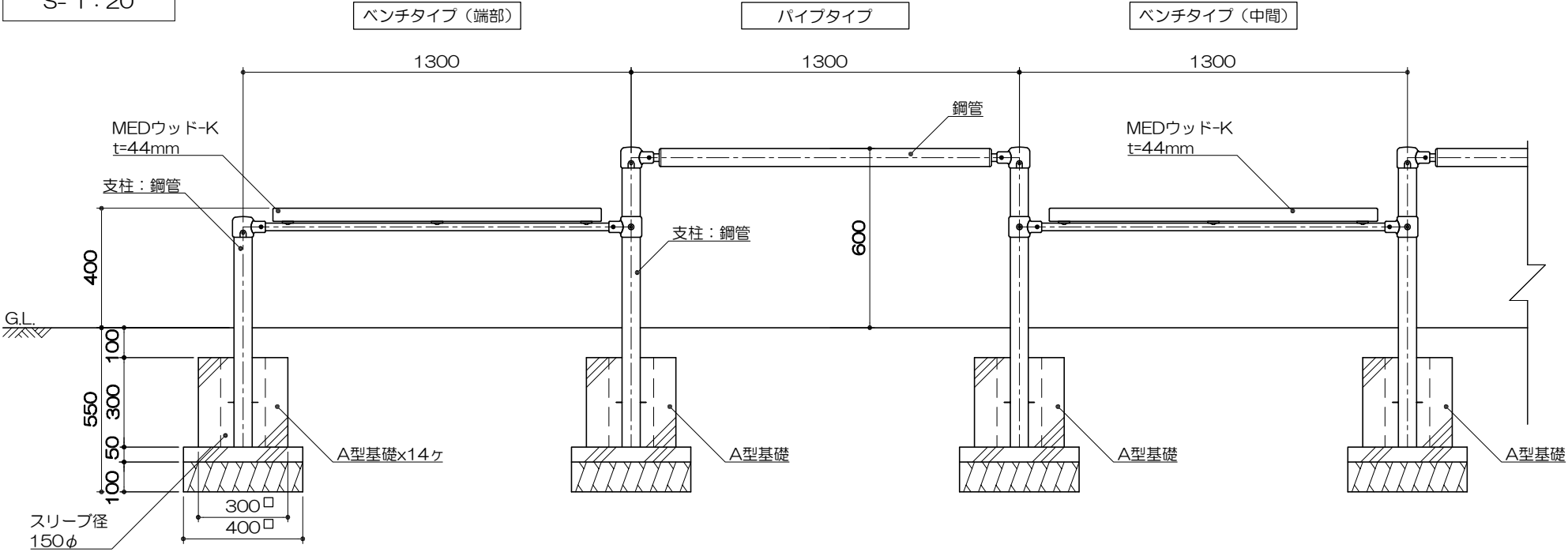
展開図 S= 1 : 20
