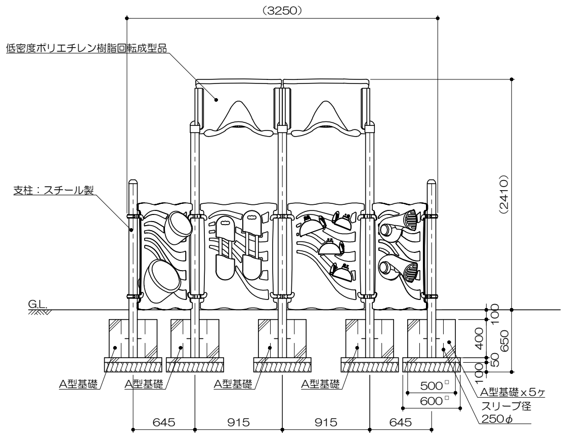
立面図 S= 1 : 40
