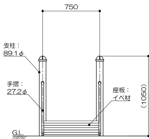
側面図 S= 1 : 30
