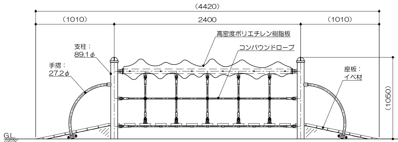
立面図 S= 1 : 30
