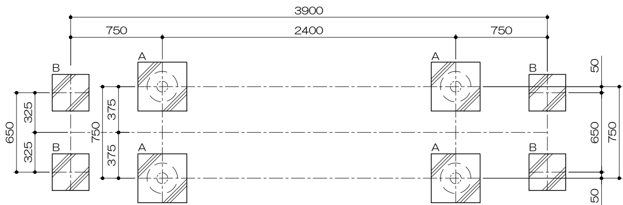
基礎平面図 S= 1 : 30
