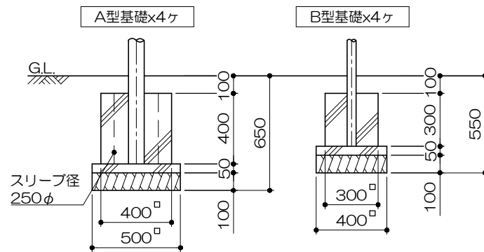
側面図 S= 1 : 30
