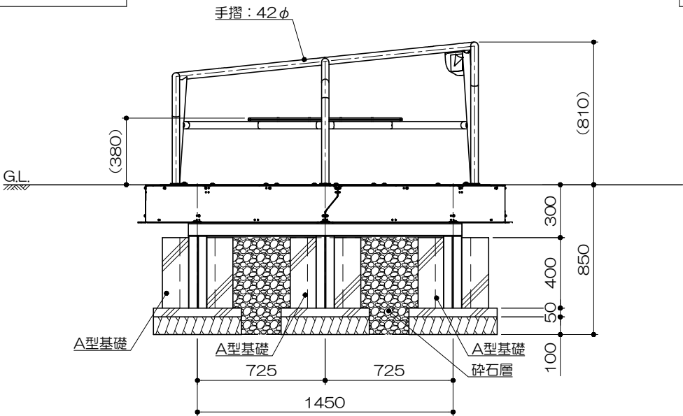
立面図 S= 1 : 30
