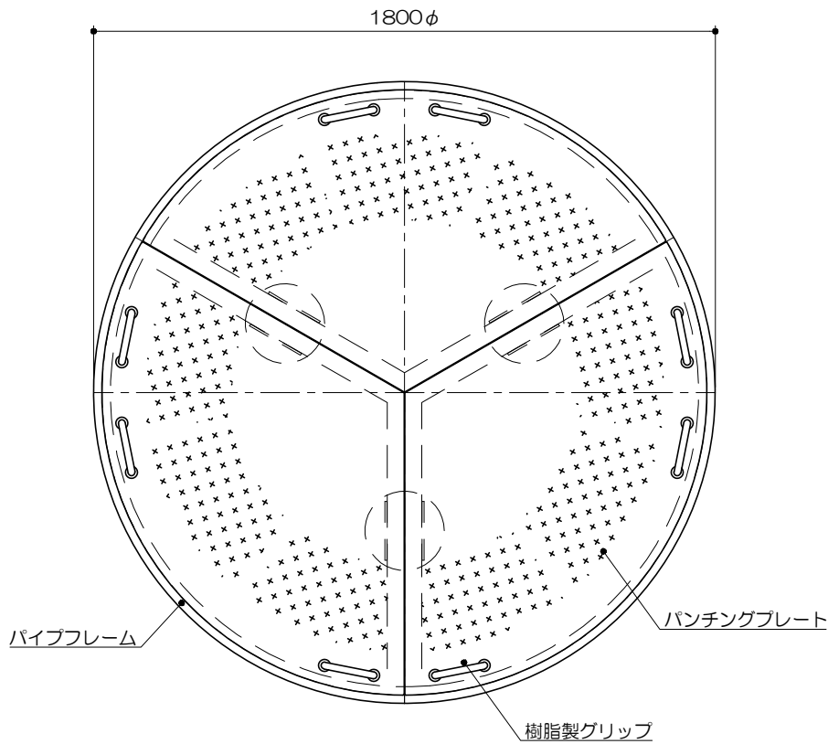
平面図 S= 1 : 20
