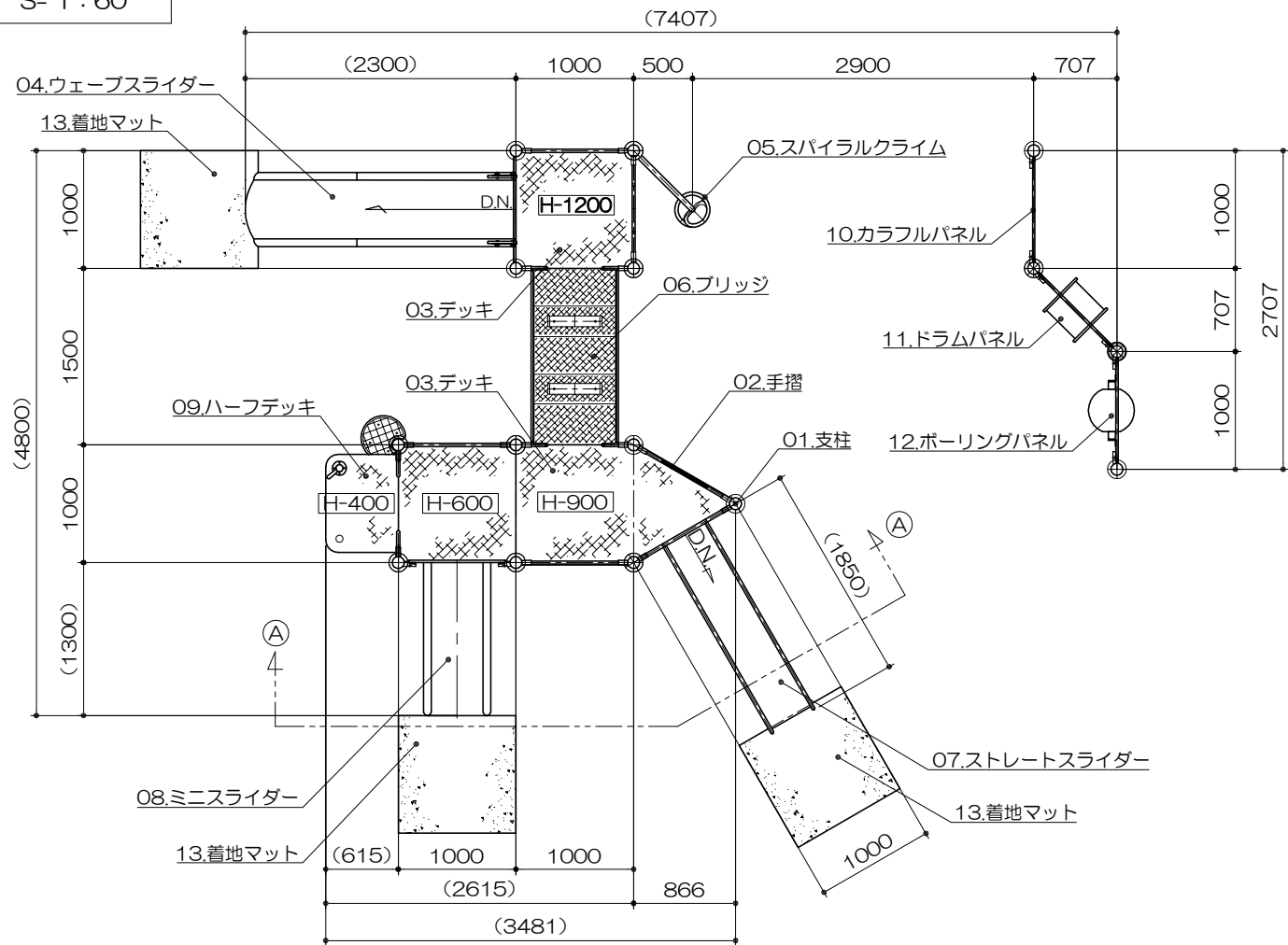
平面図 S= 1 : 60
