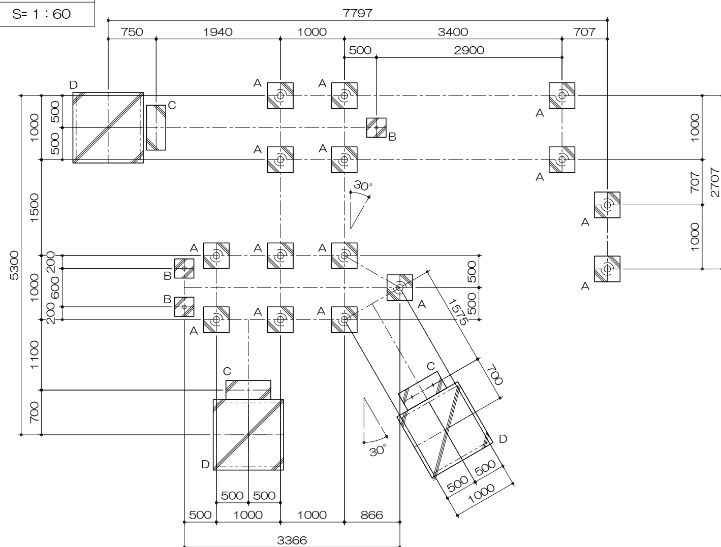
基礎平面図
