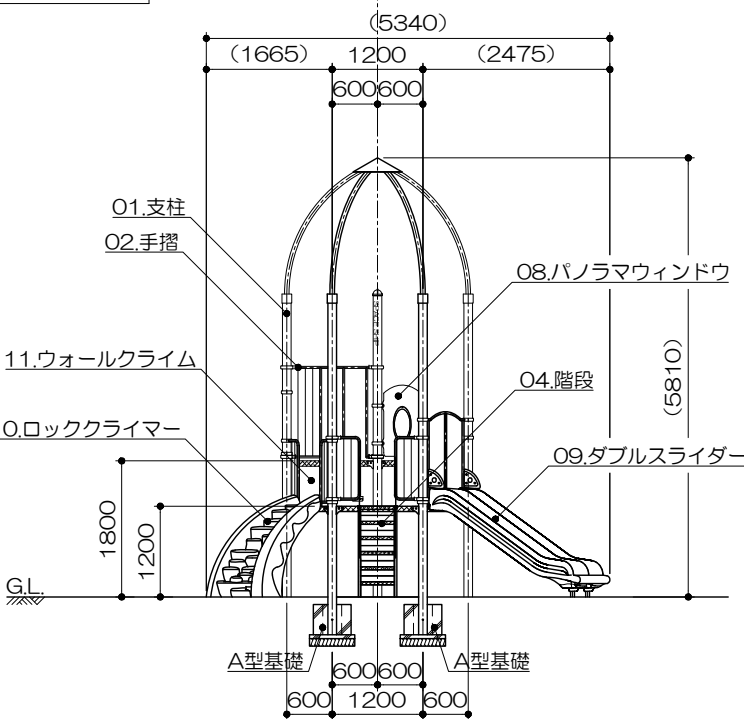
側面図 S= 1 : 100
