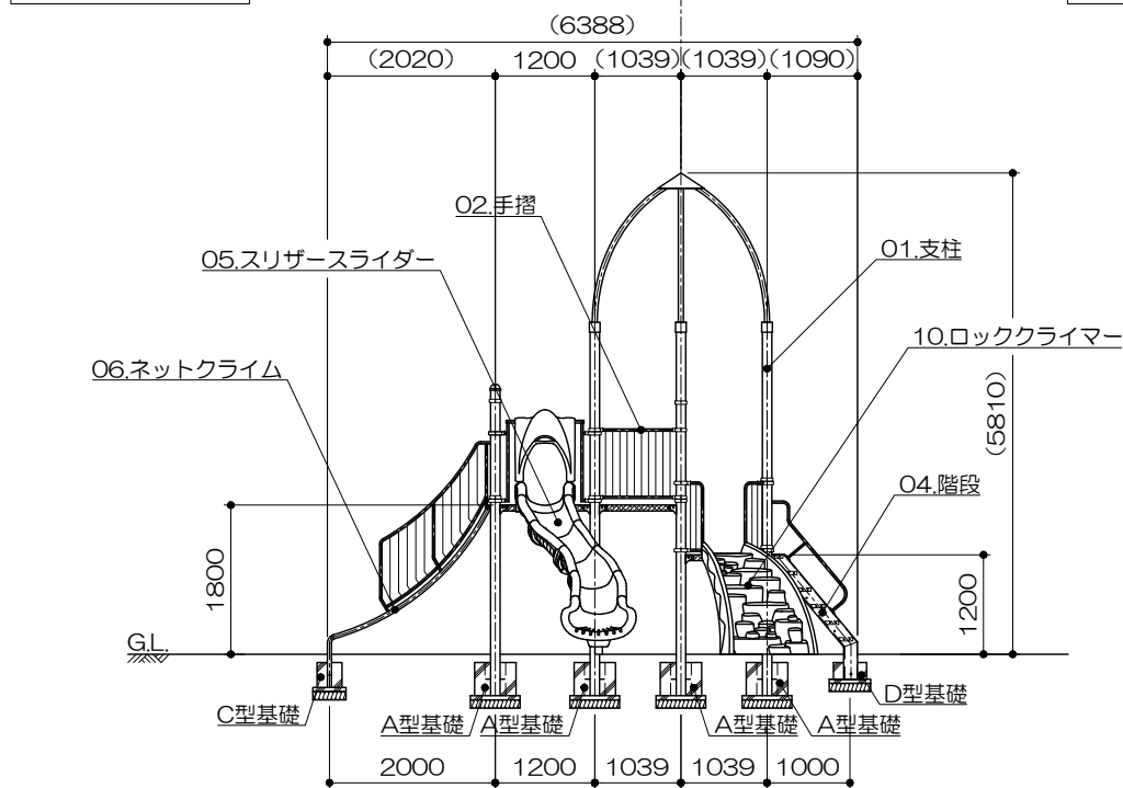
立面図 S= 1 : 100
