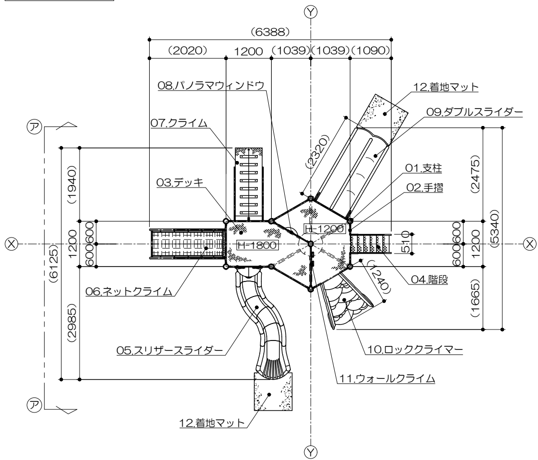
平面図 S= 1 : 100
