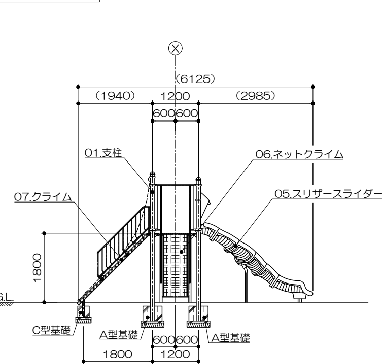
ア-ア 矢視図 S= 1 : 100
