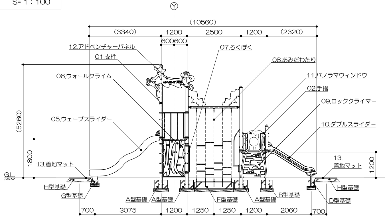
立面図 S= 1 : 100
