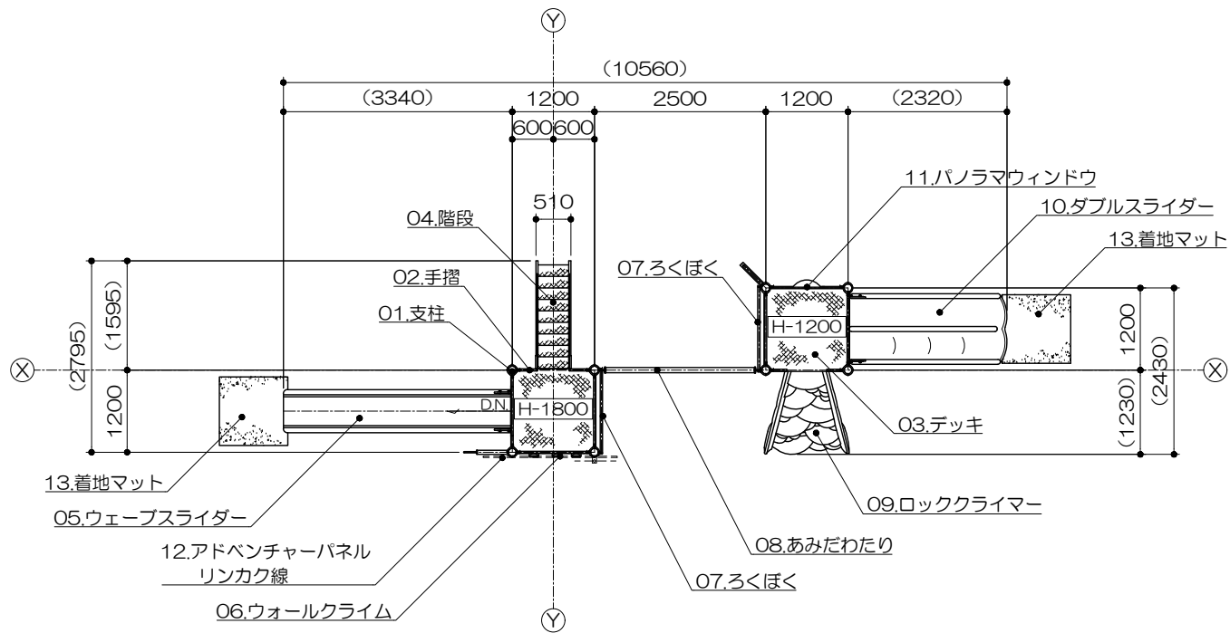
平面図 S= 1 : 100
