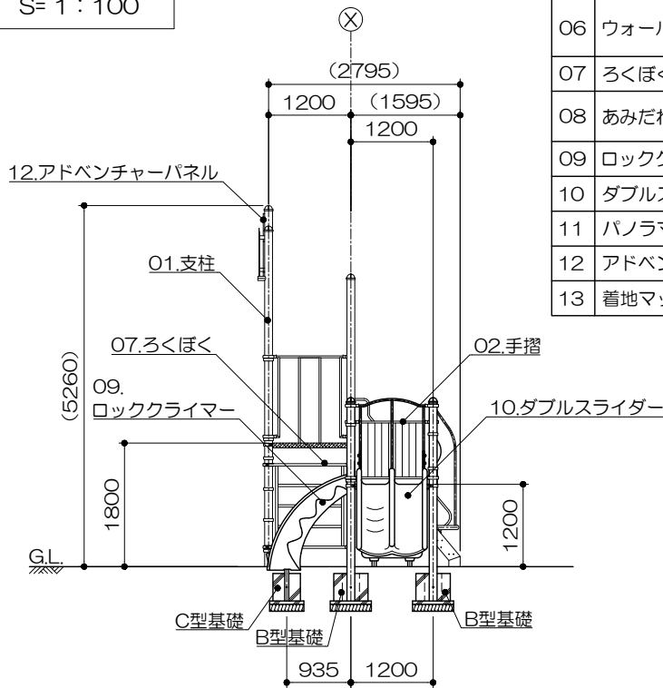
側面図 S= 1 : 100
