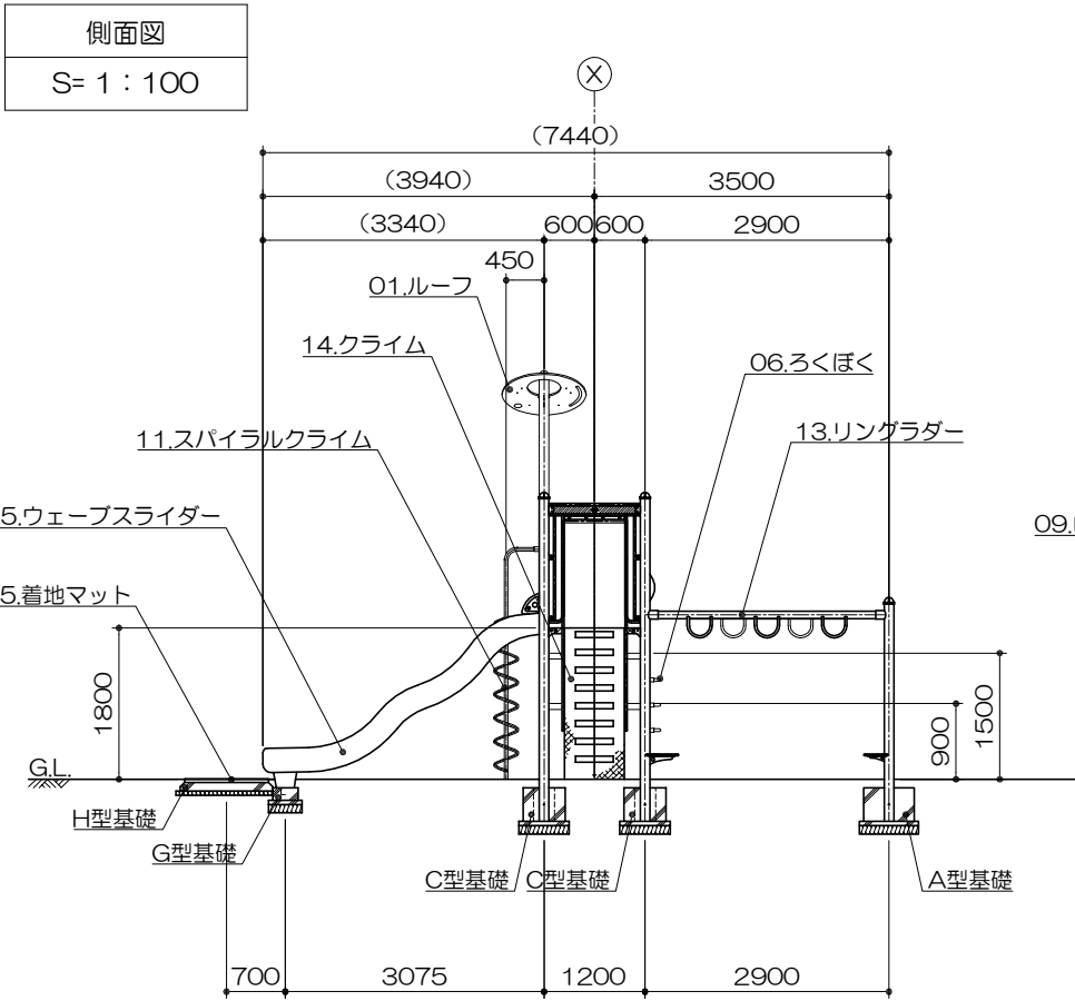
A-A立面図 S= 1 : 100
