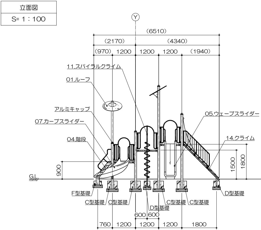
側面図 S= 1 : 100
