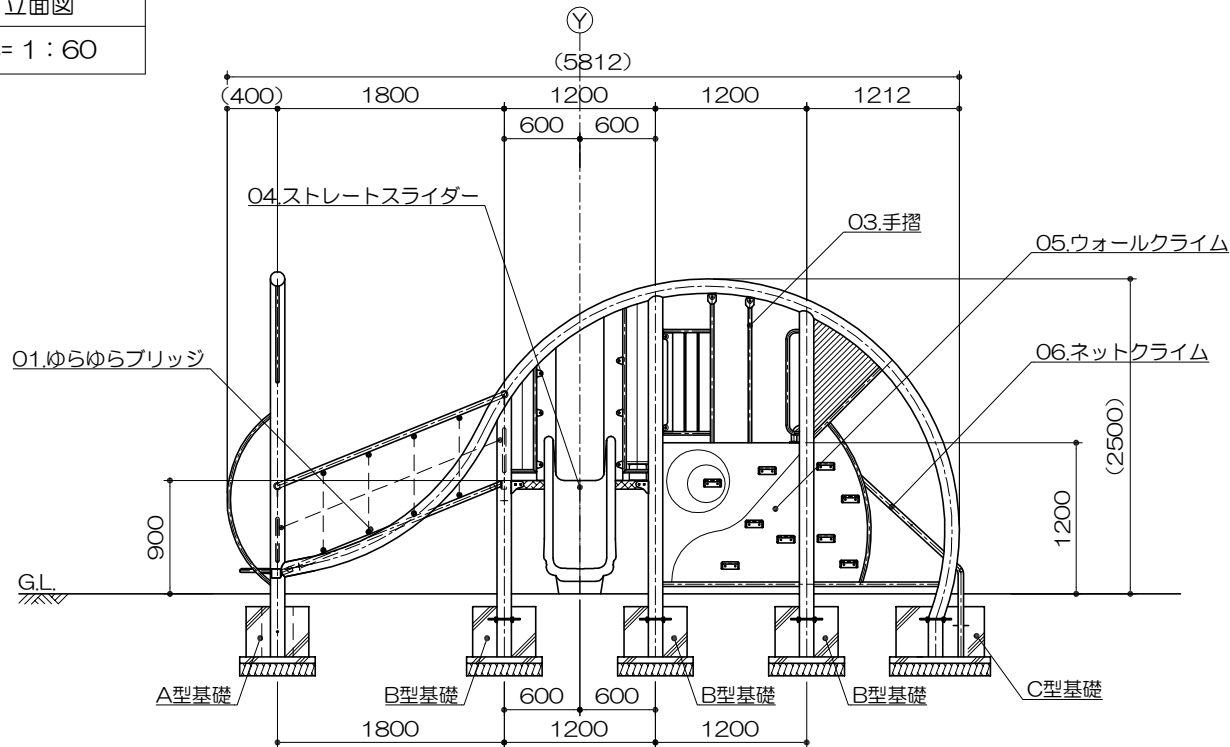
側面図 S= 1 : 60
