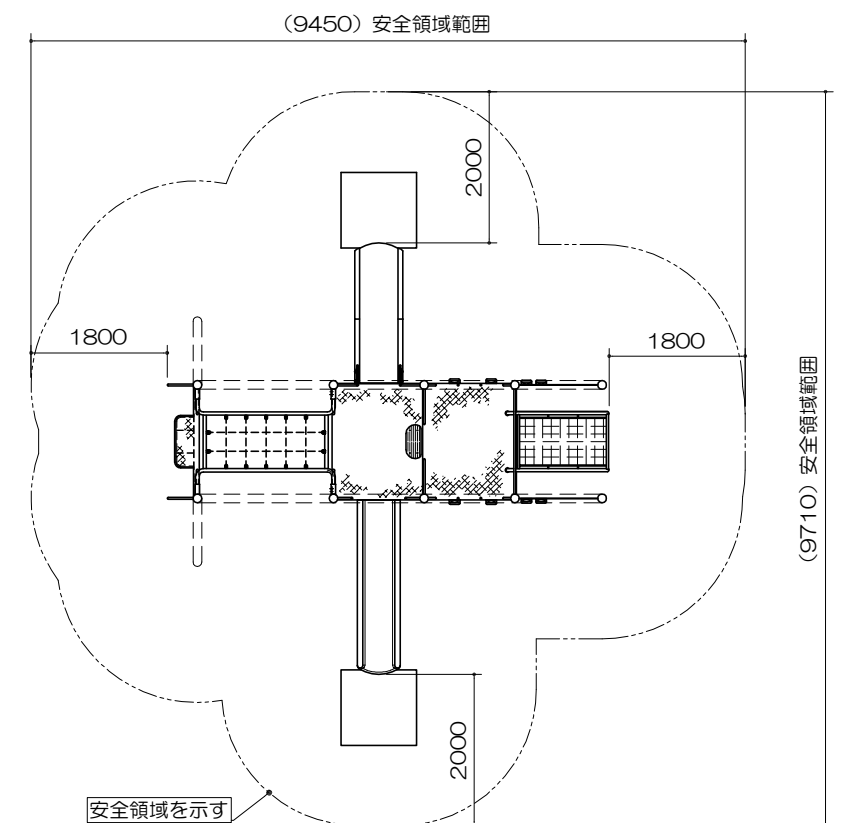
安全領域範囲 S= 1 : 100
