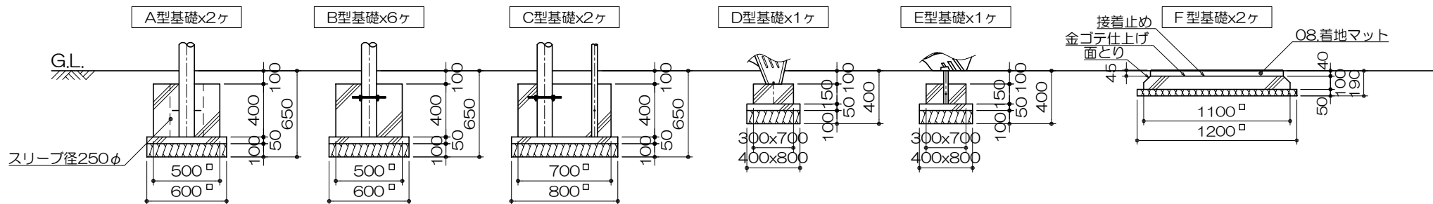
基礎リスト S= 1 : 40
