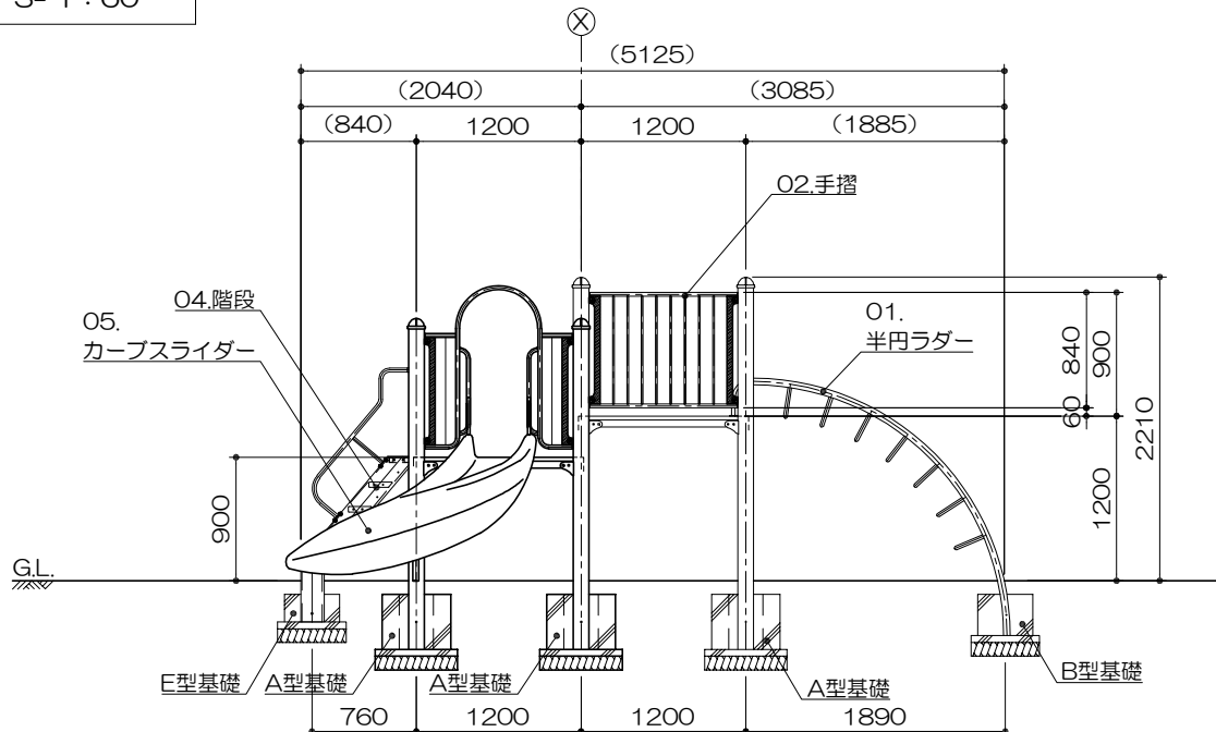
S= 1 : 60
