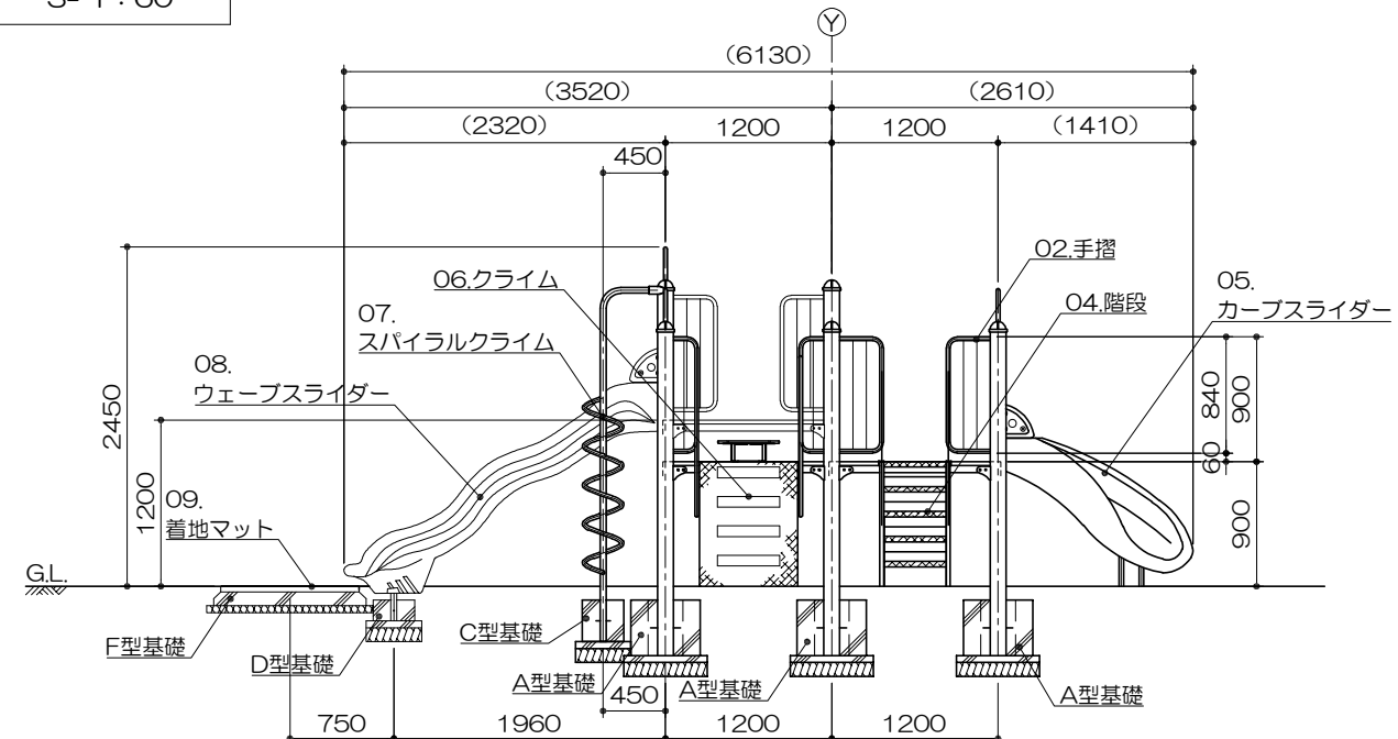
S= 1 : 60
