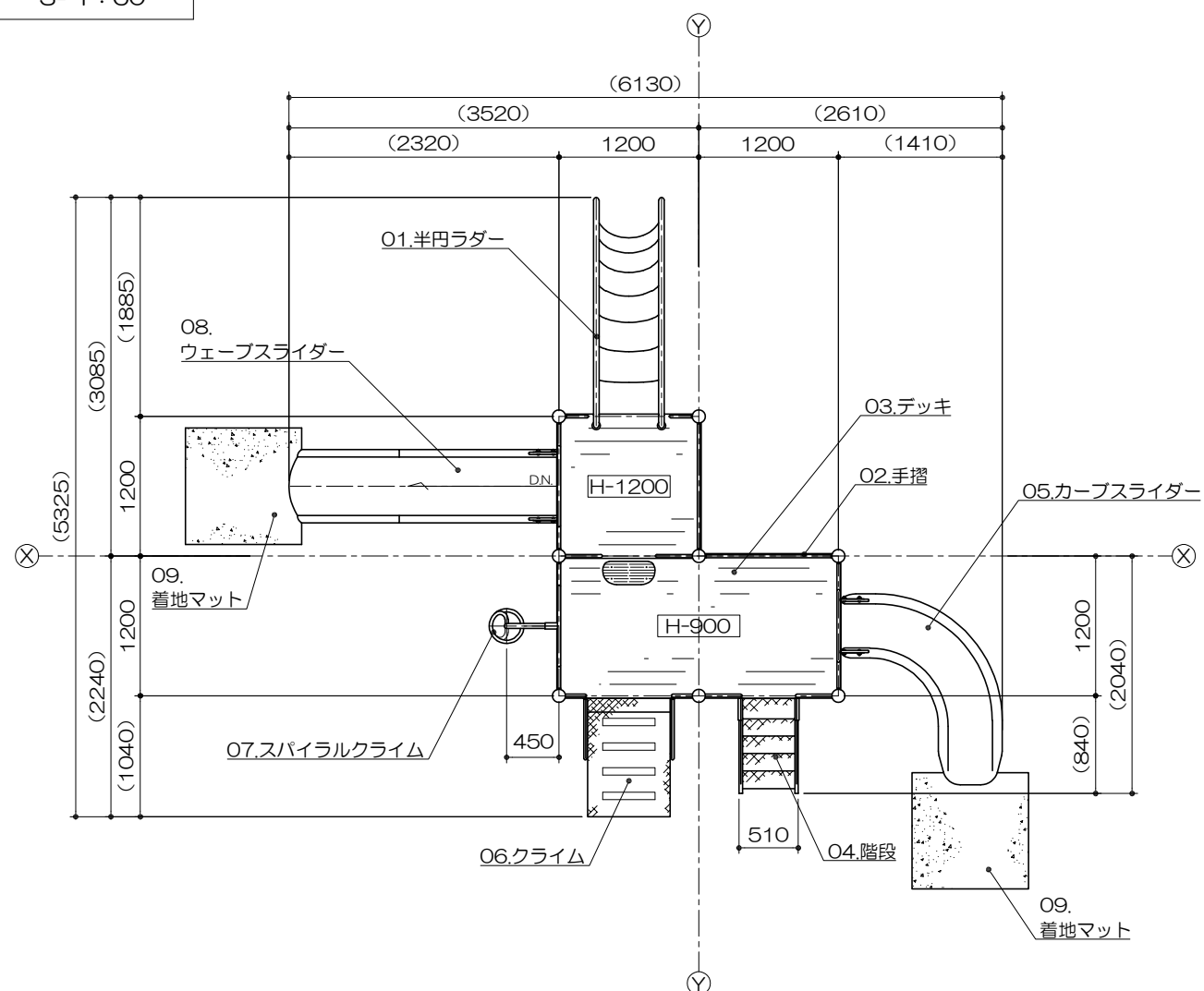
S= 1 : 60
