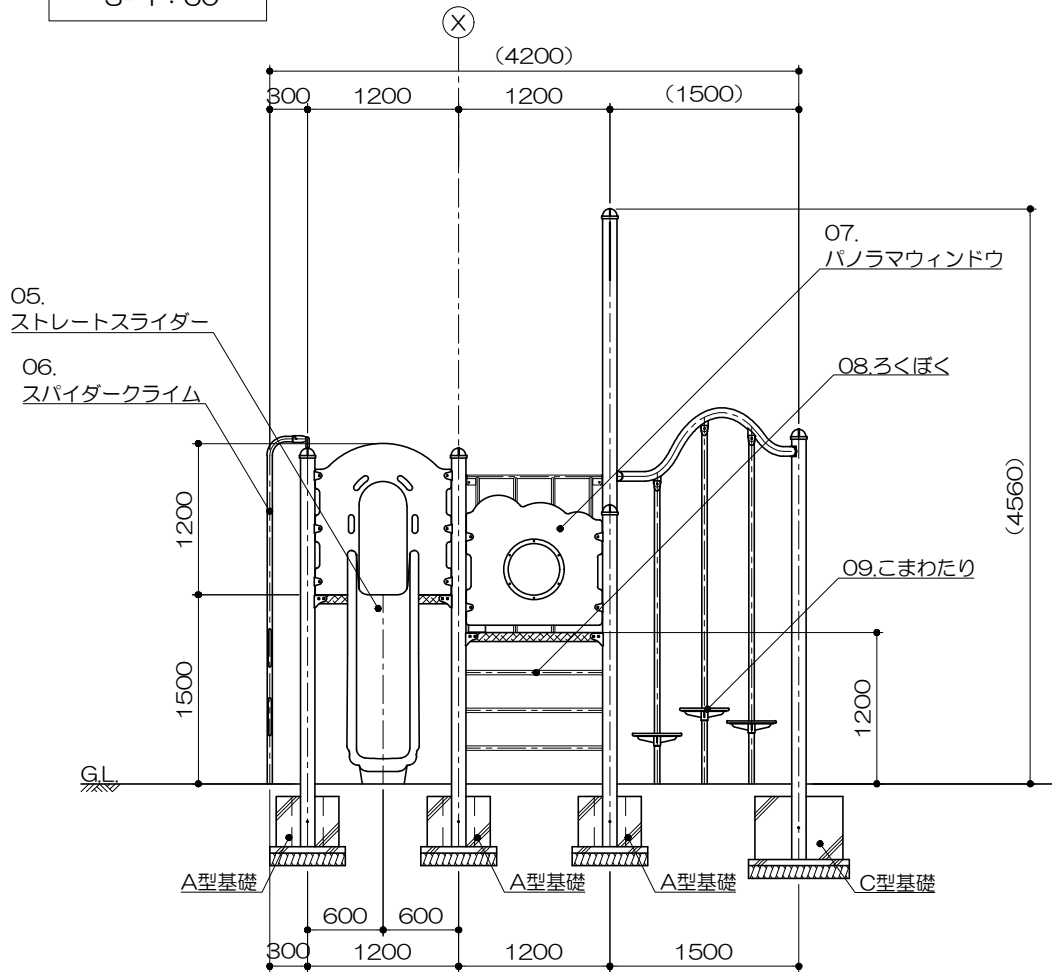
側面図 S= 1 : 60
