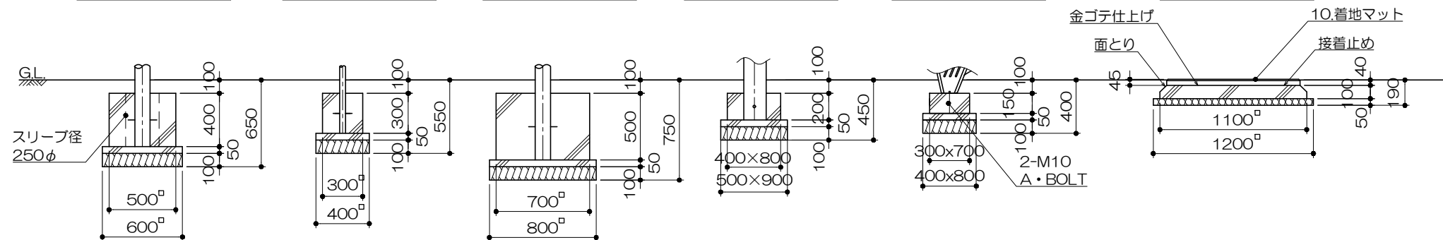
A型基礎x6ヶ
