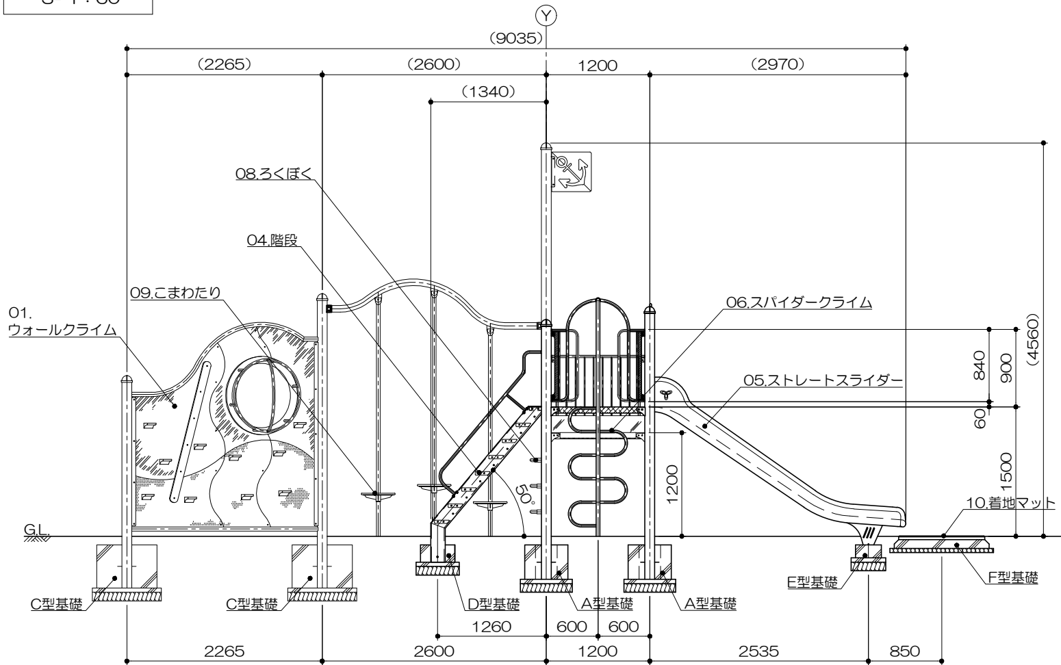
立面図 S= 1 : 60
