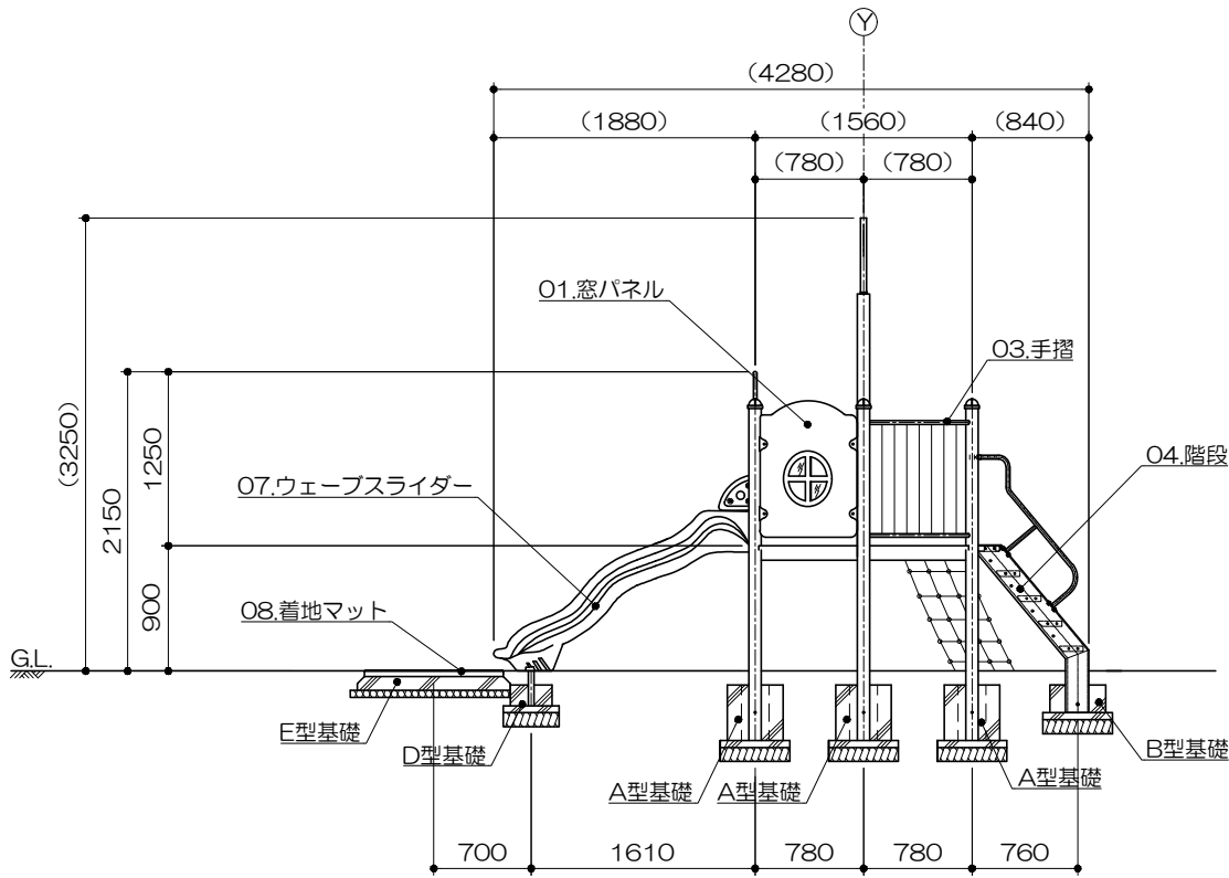
側面図 S= 1 : 60
