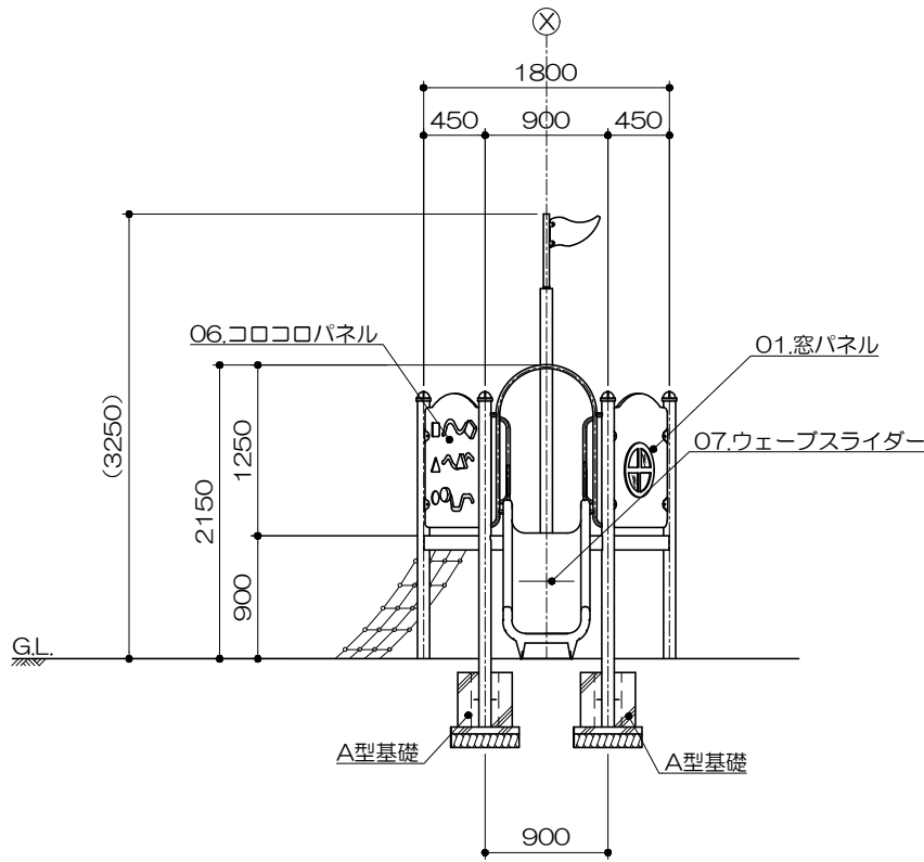
立面図 S= 1 : 60
