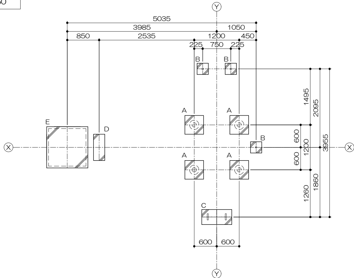
基礎平面図 S= 1 : 60
