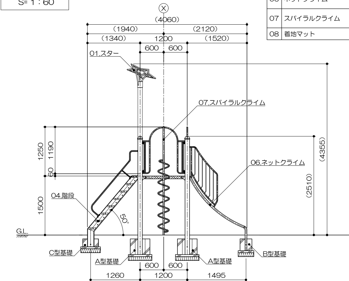
側面図 S= 1 : 60
