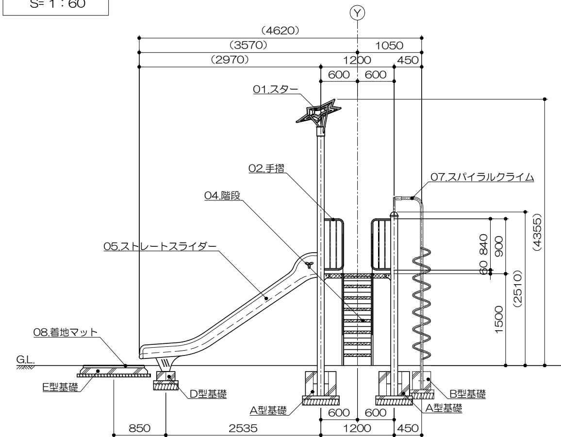
立面図 S= 1 : 60
