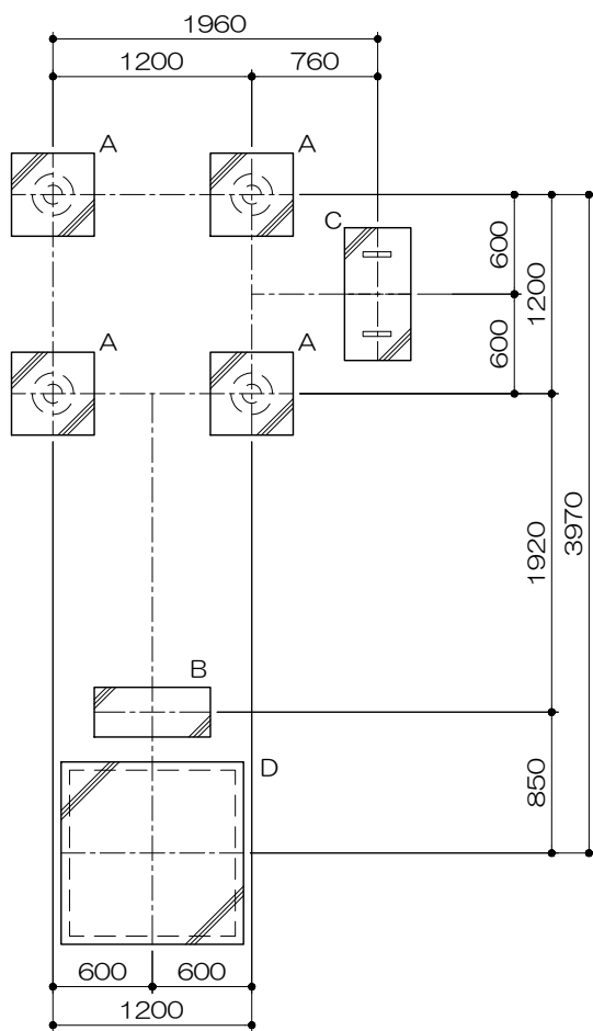
基礎平面図 S= 1 : 50
