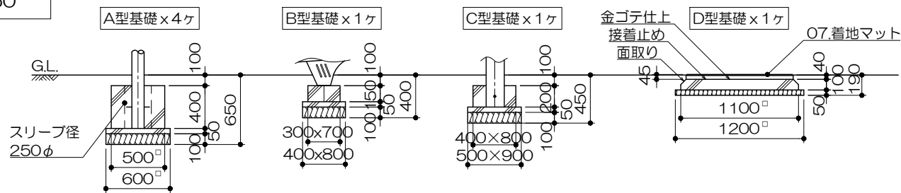
基礎リスト S= 1 : 50
