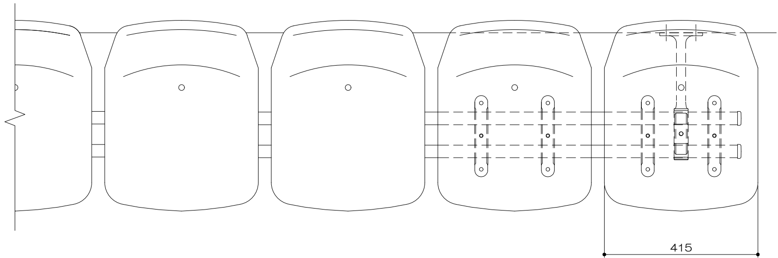
立面図 S= 1 : 10
