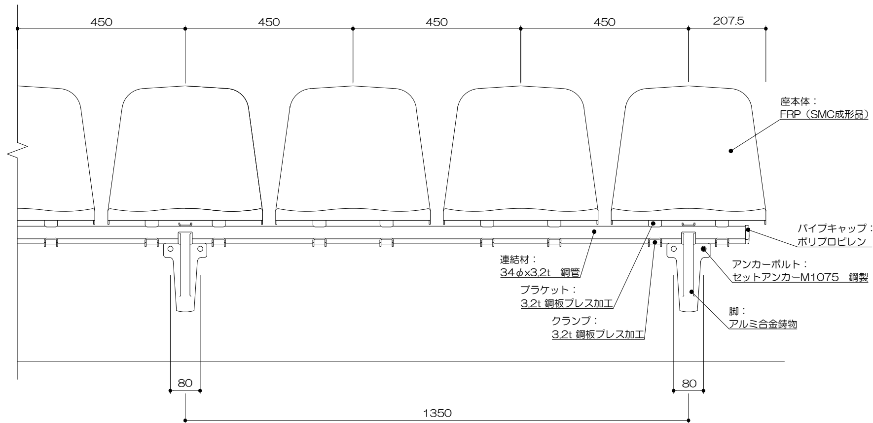
立面図 S= 1 : 10
