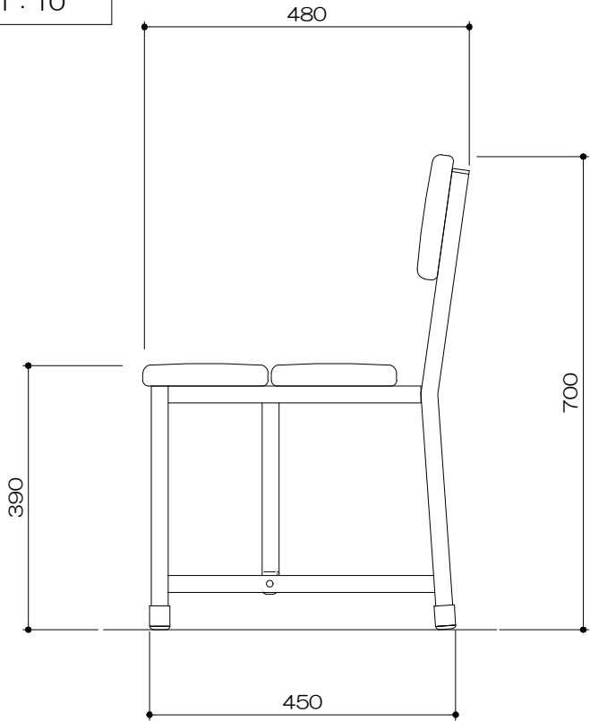
側面図 S= 1 : 10
