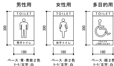
ピクトサイン詳細図 Scale 1:20 アルミ複合板-180x300xt3.0 絵柄：インクジェット印刷(UVフィルム貼り)
