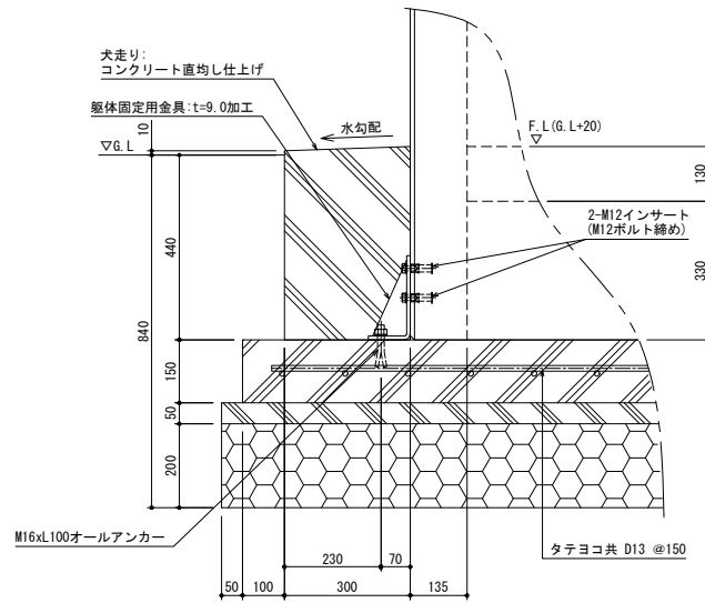
基礎部断面 詳細図 (a-a) Scale 1:20
