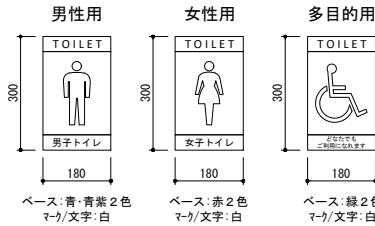
ピクトサイン詳細図
