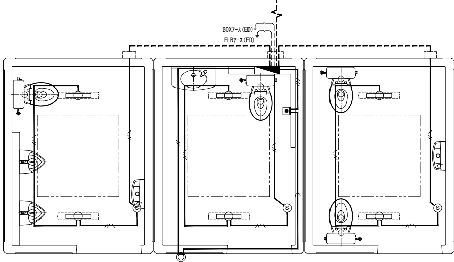
「電気」系統 参考図
