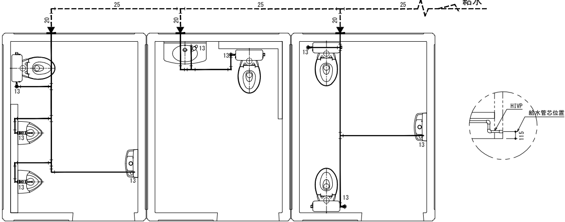
「給水」系統 参考図
