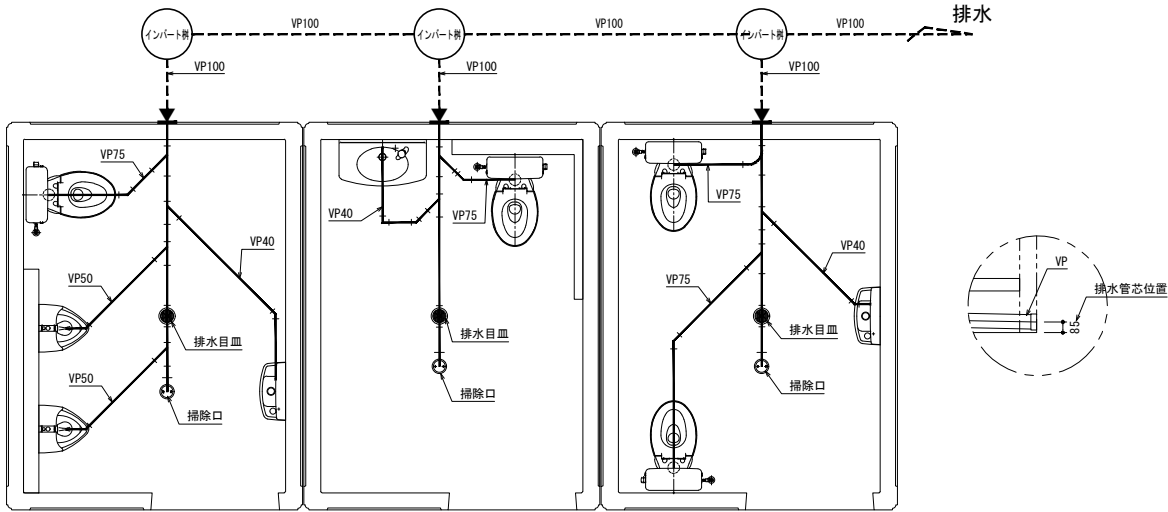
「排水」系統 参考図
