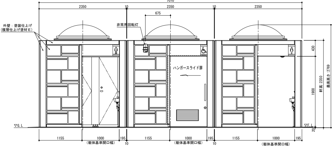
正面図
