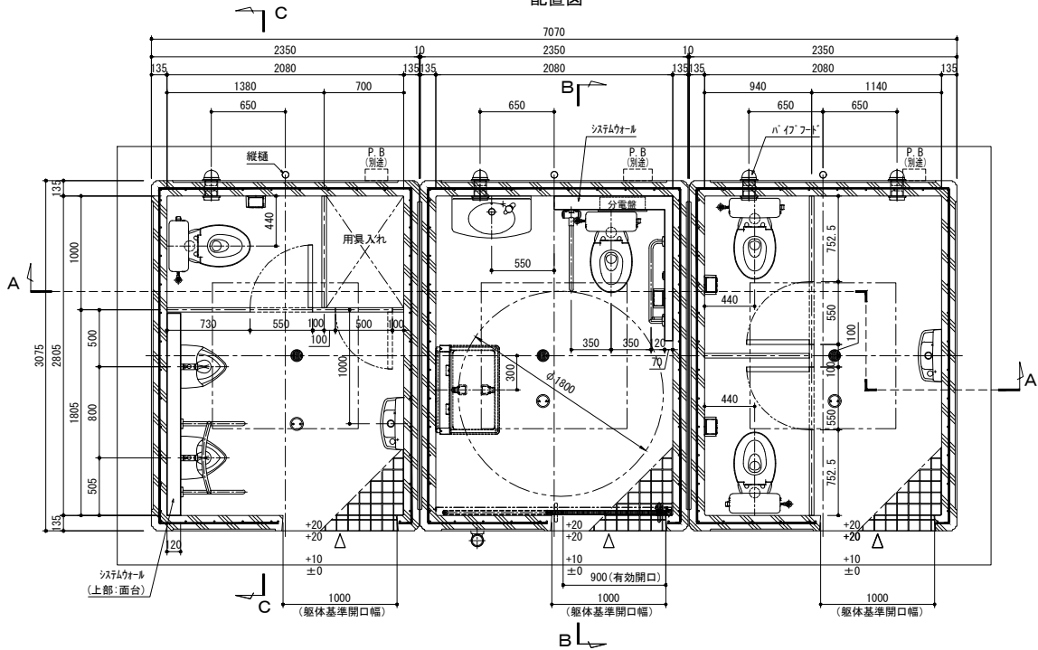
配置図
