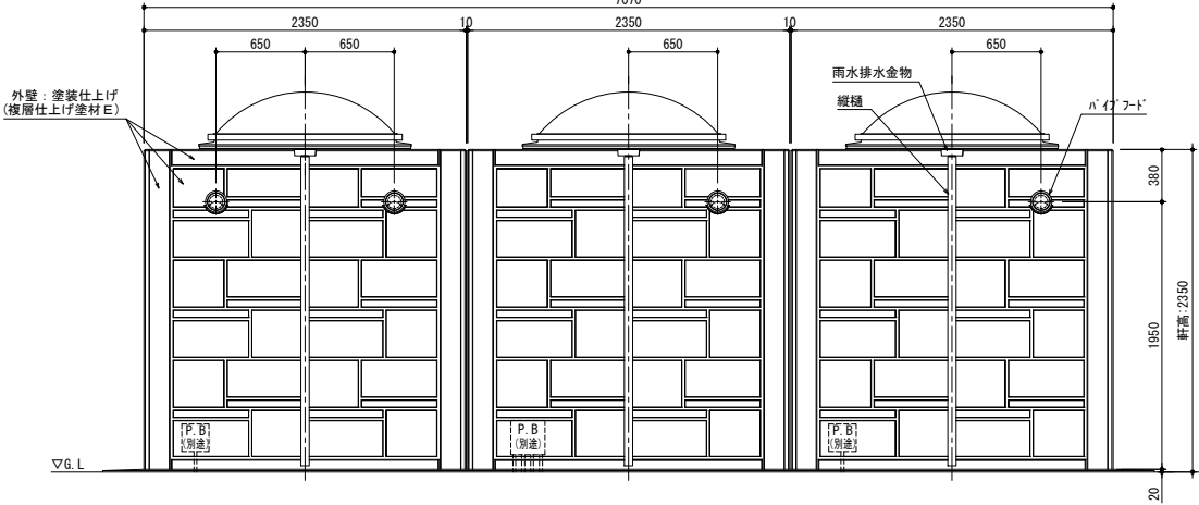
背面図
