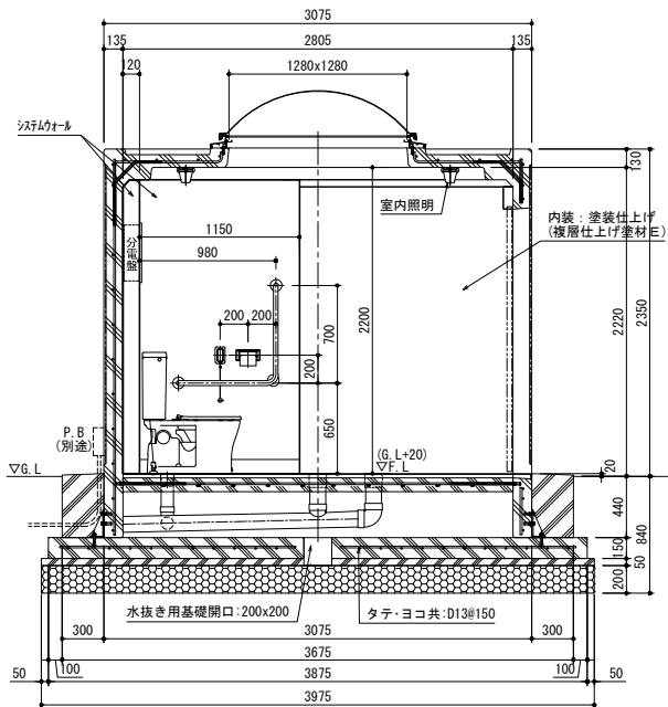
B-B 断面図
