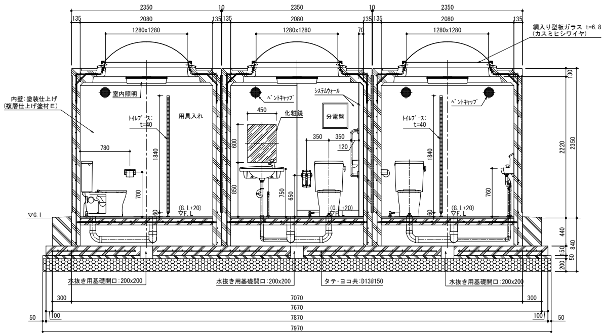
A-A 断面図
