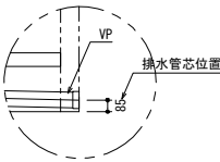
排水管接続口詳細図
