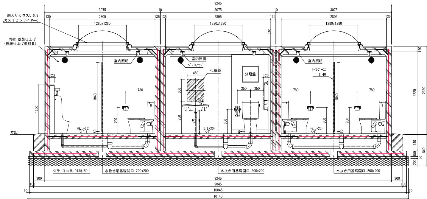
A-A 断面図
