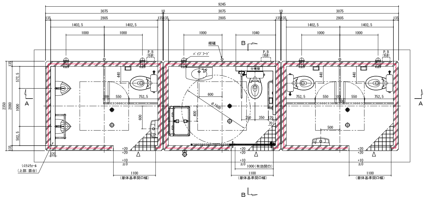
配置図
