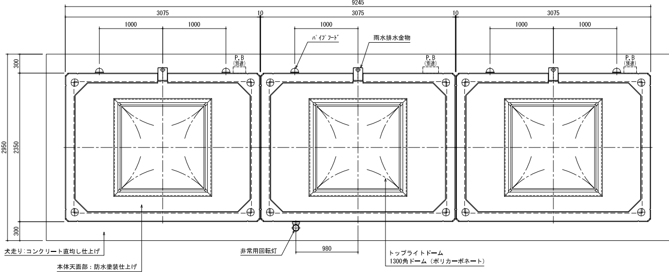
平面図
