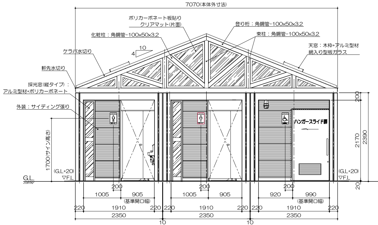
正面図 S= 1 : 60
