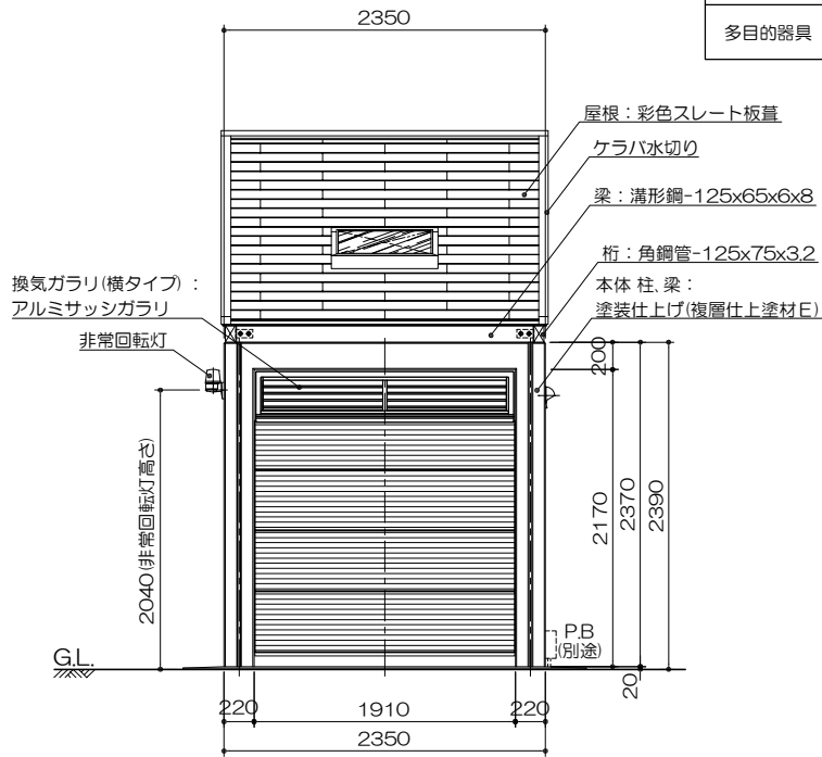
側面図 S= 1 : 60
