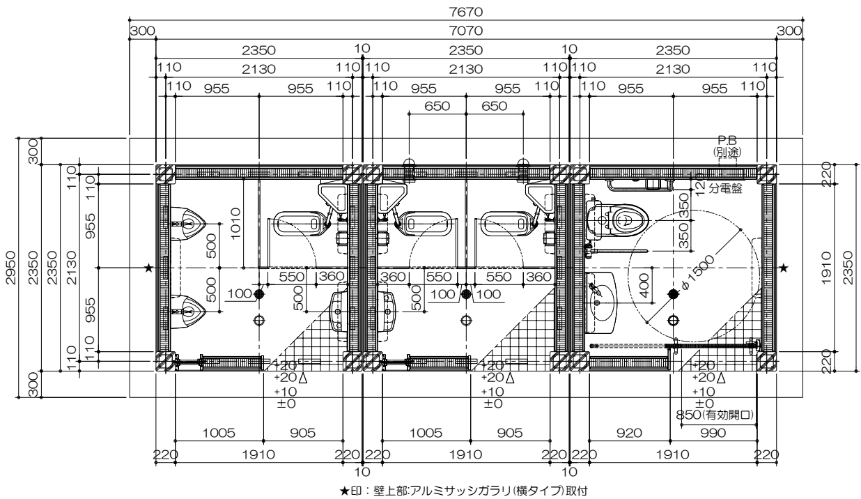
平面図 S= 1 : 60
