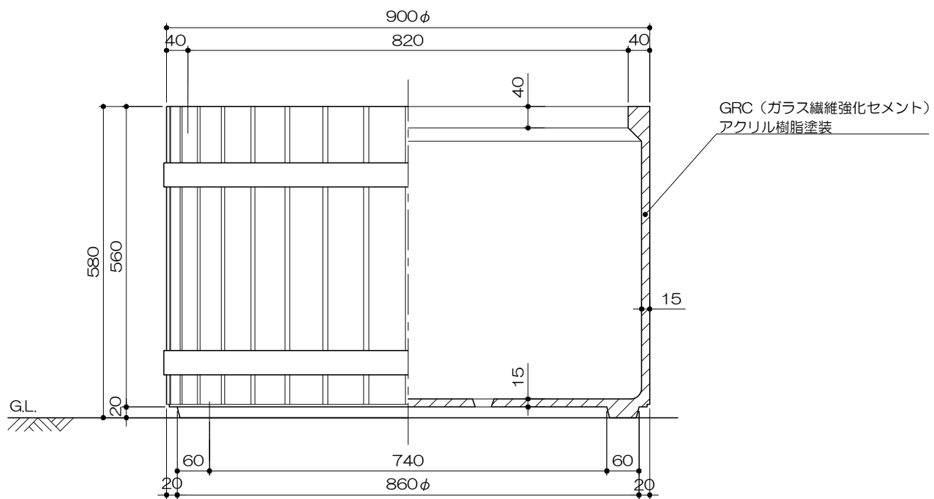
立面図 S= 1 : 10
