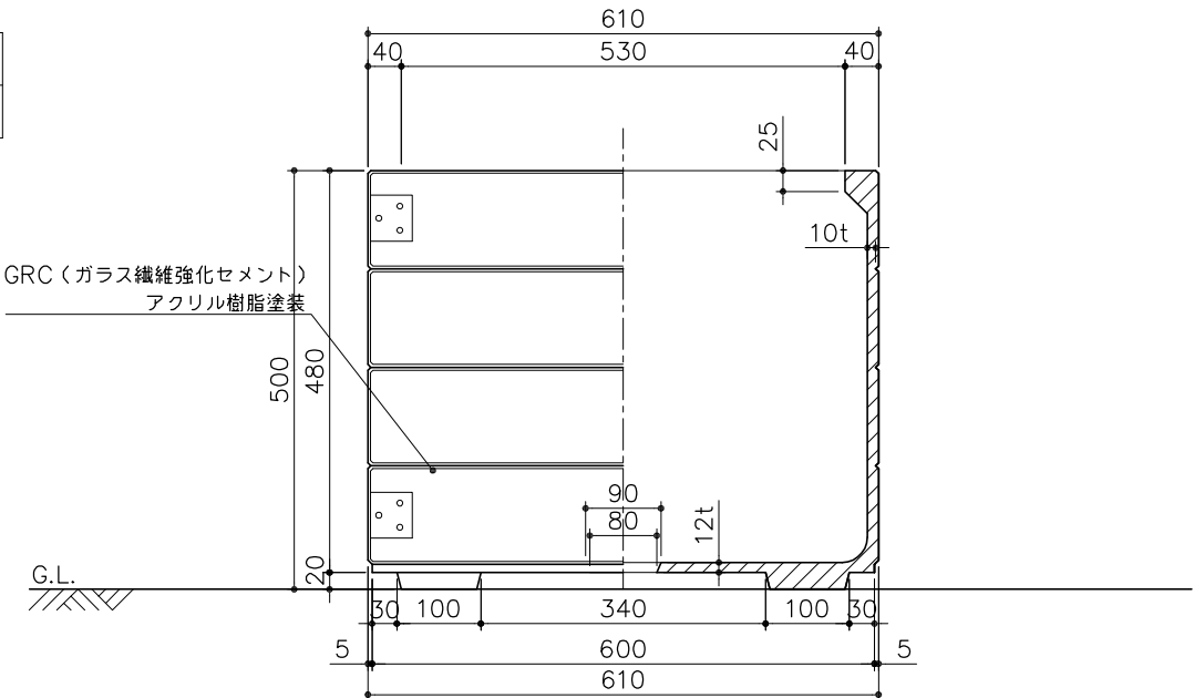
立・断面図 S= 1:10
