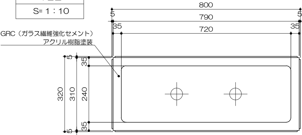
立・断面図 S= 1 : 10
