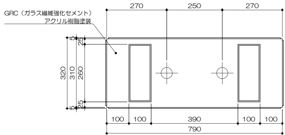
底面図 S= 1 : 10
