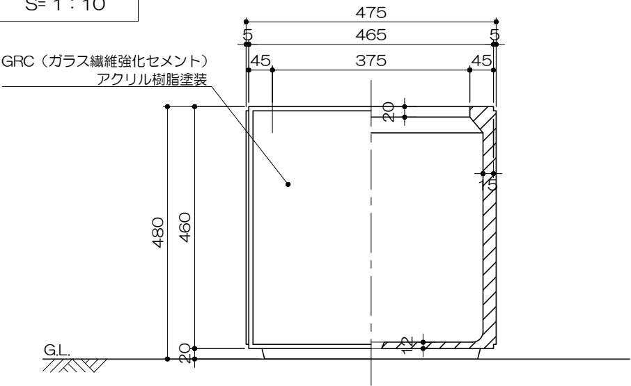
側・断面図 S= 1 : 10
