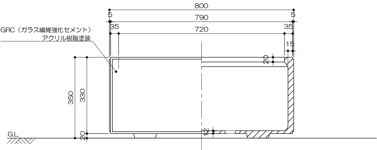
立・断面図 S= 1 : 10
