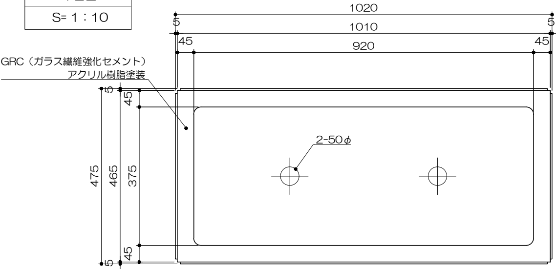
立・断面図 S= 1 : 10
