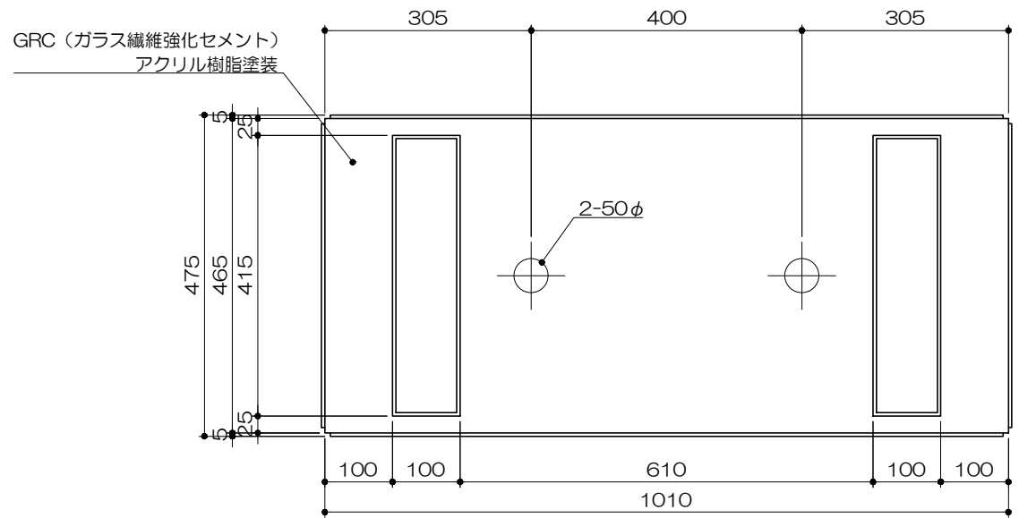
底面図 S= 1 : 10
