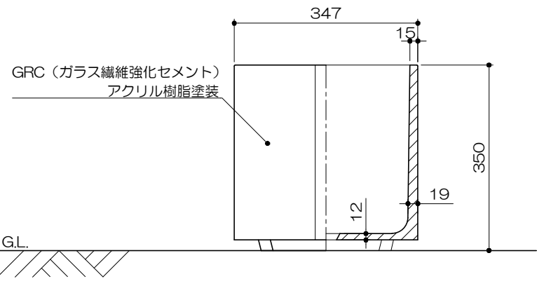
側・断面図 S= 1 : 10
