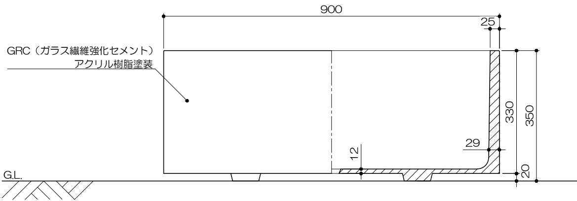
立・断面図 S= 1 : 10
