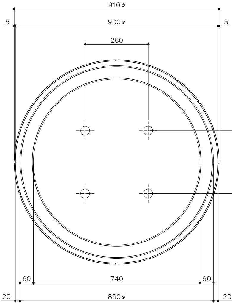
底面図 S= 1 : 10
