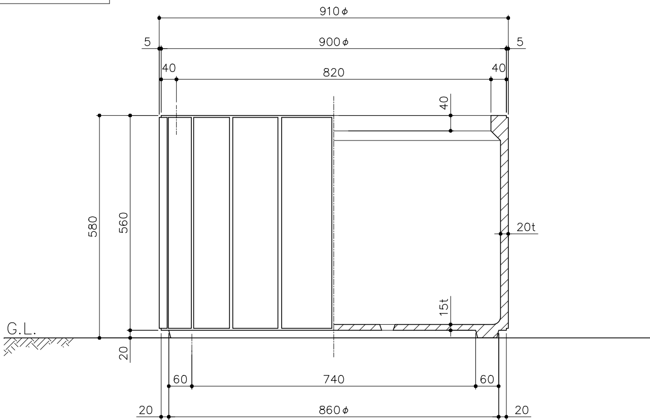
立・断面図 S= 1 : 10
