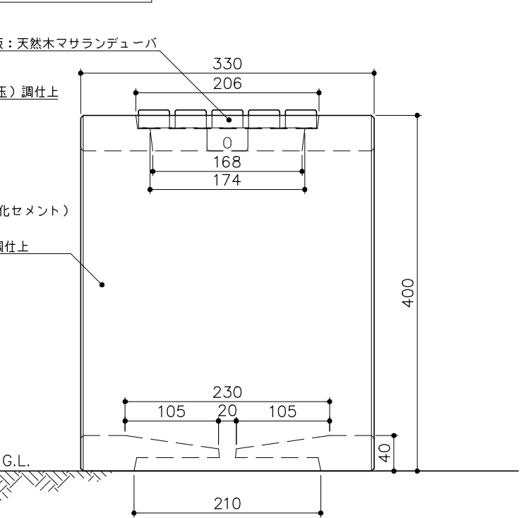
側面図 S= 1：6
