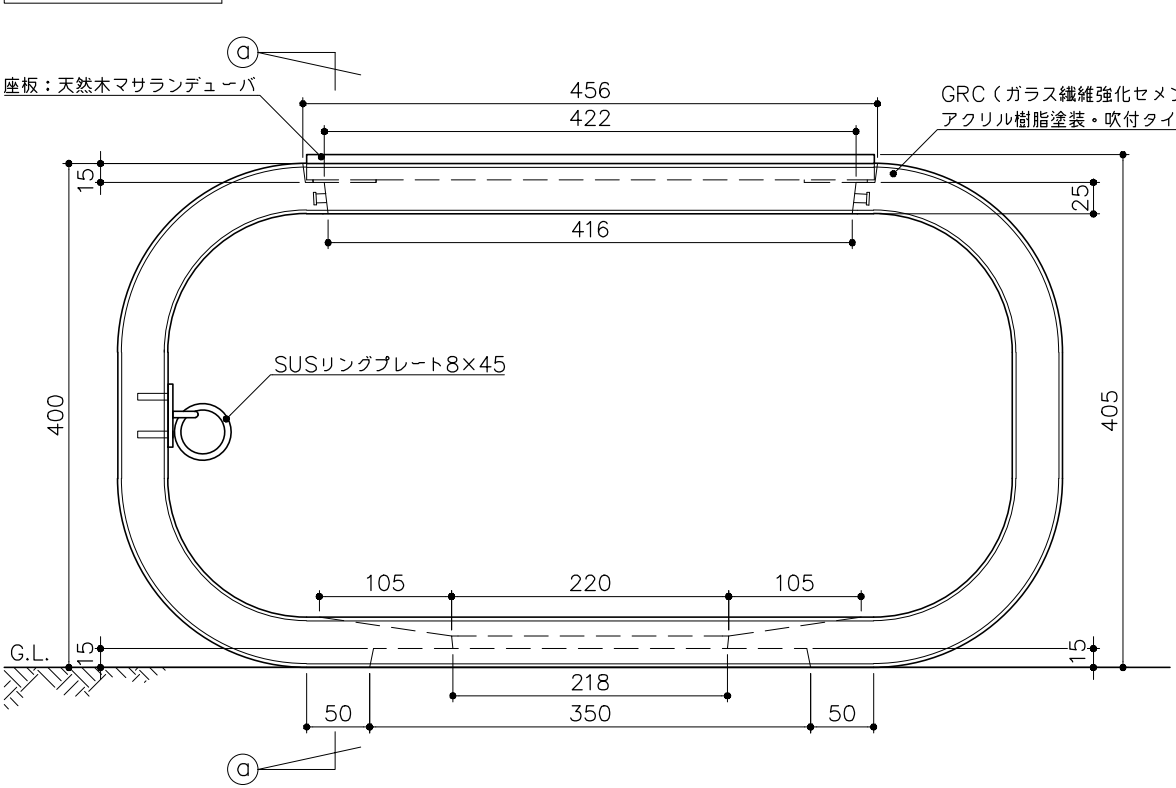
立面図 S= 1：6
