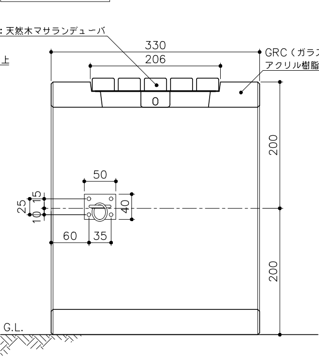
α-α断面図 S= 1：6
