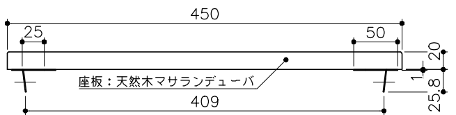
側面図 S= 1：6
