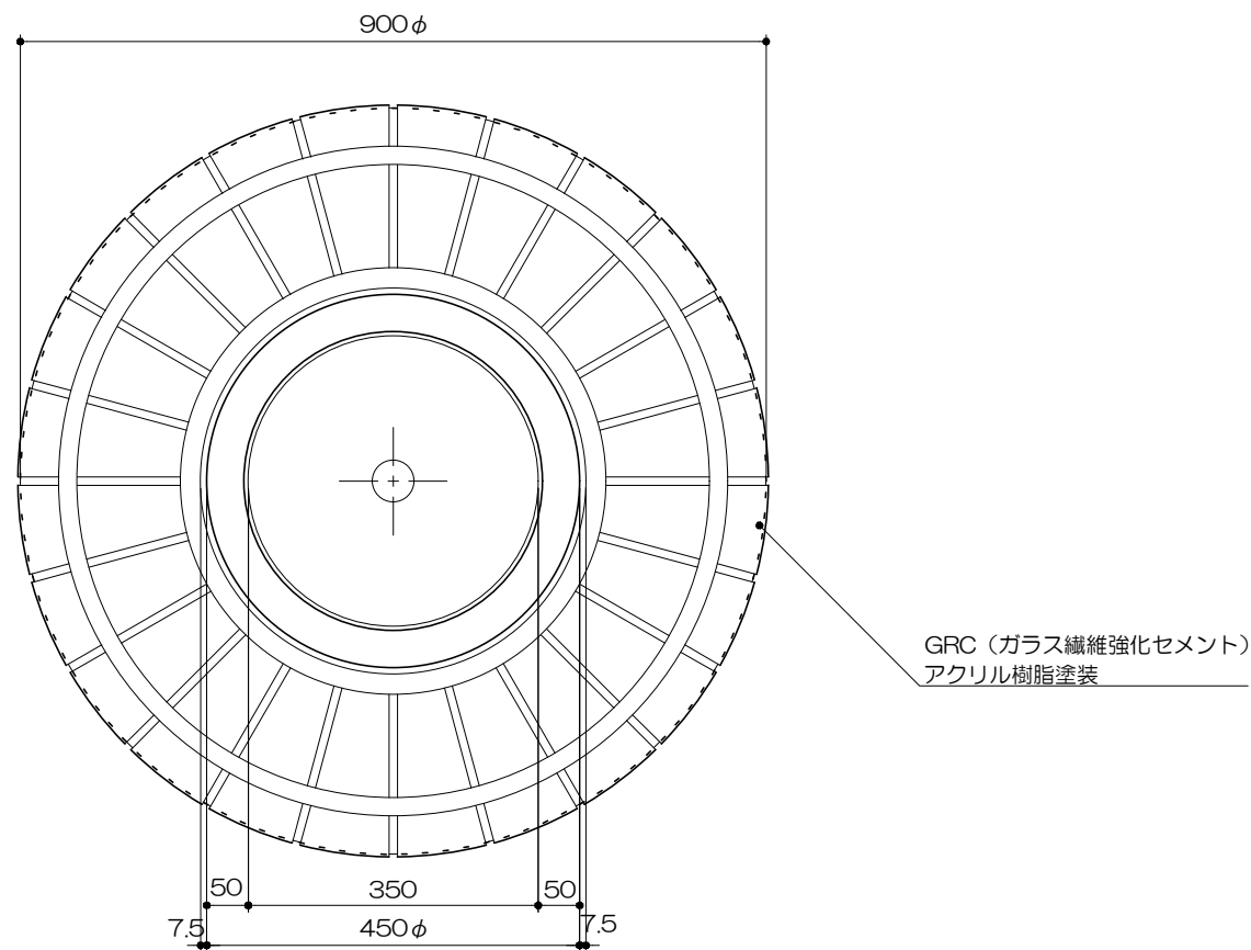
底面図 S= 1 : 10
