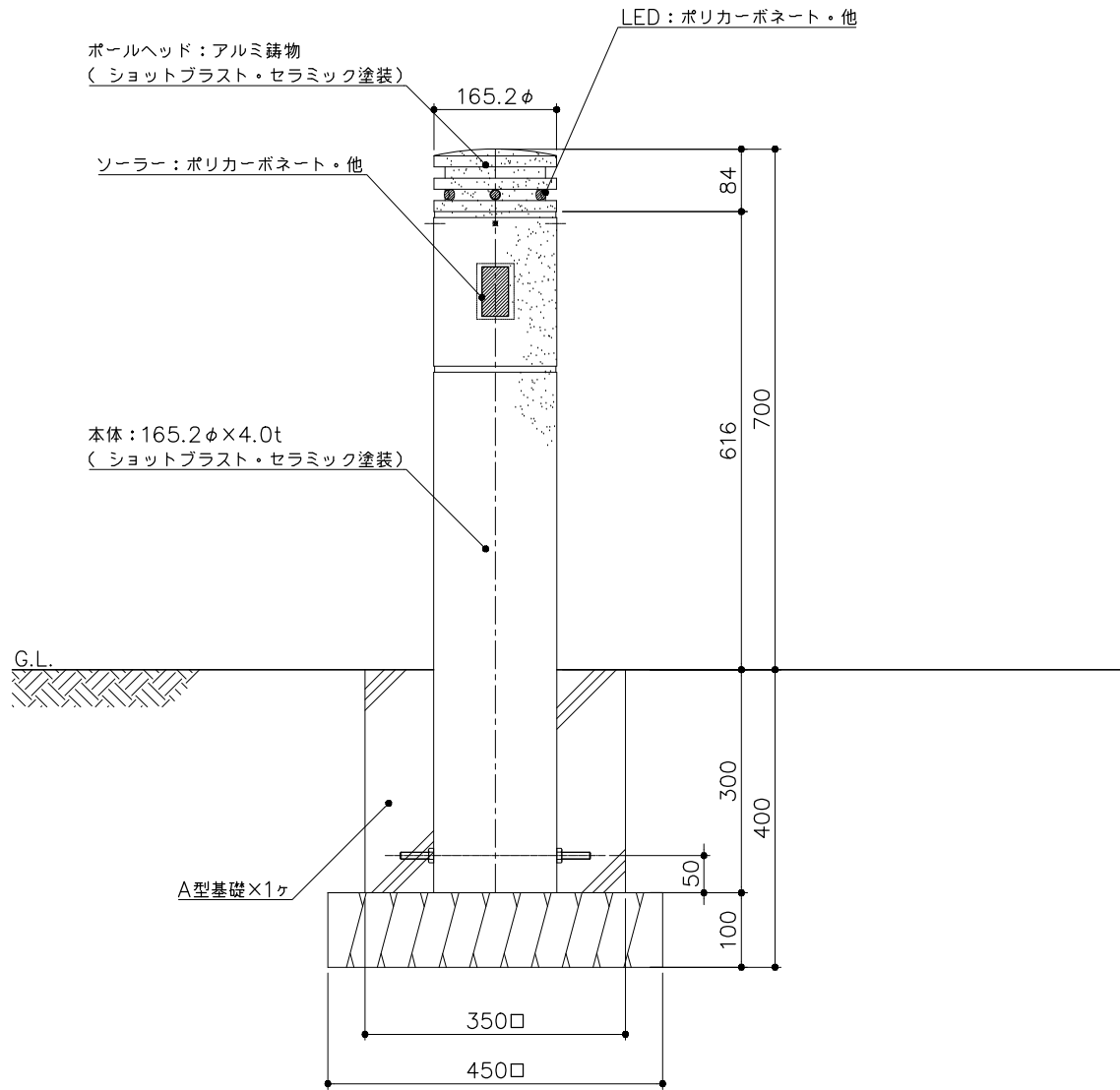
立面図 S= 1：10
