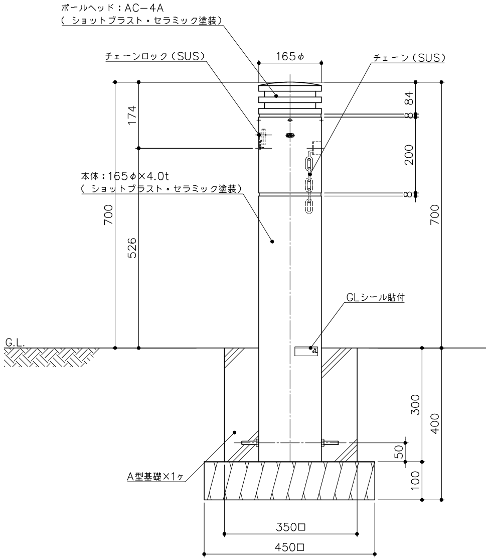
立面図 S= 1 : 10
