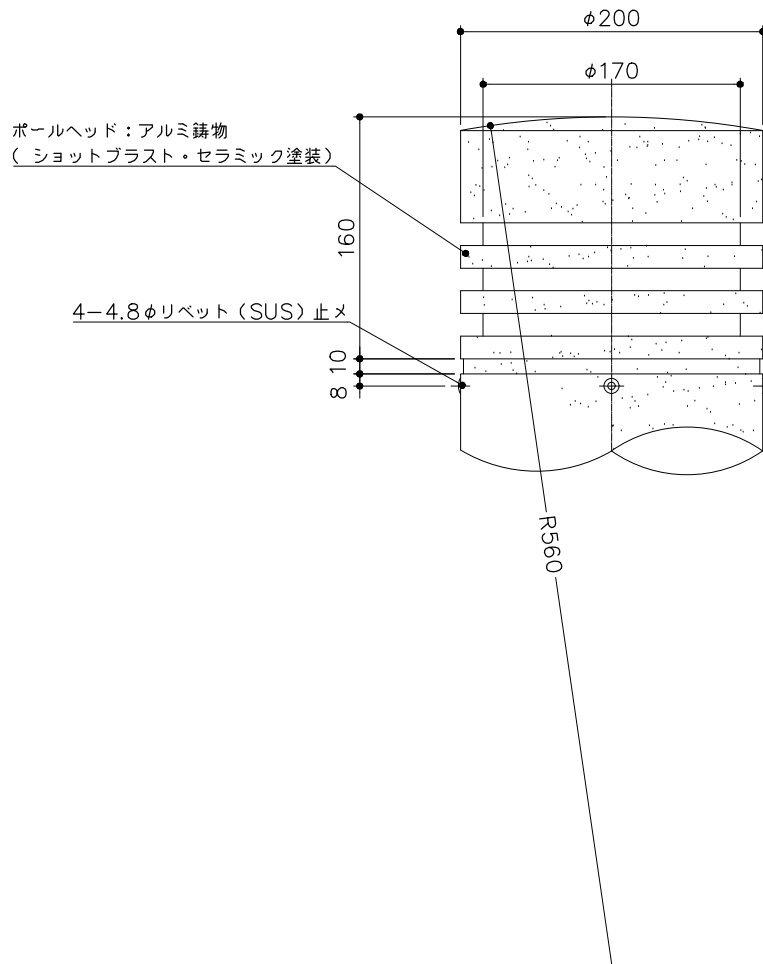
ボールヘッド詳細図 S= 1：5
