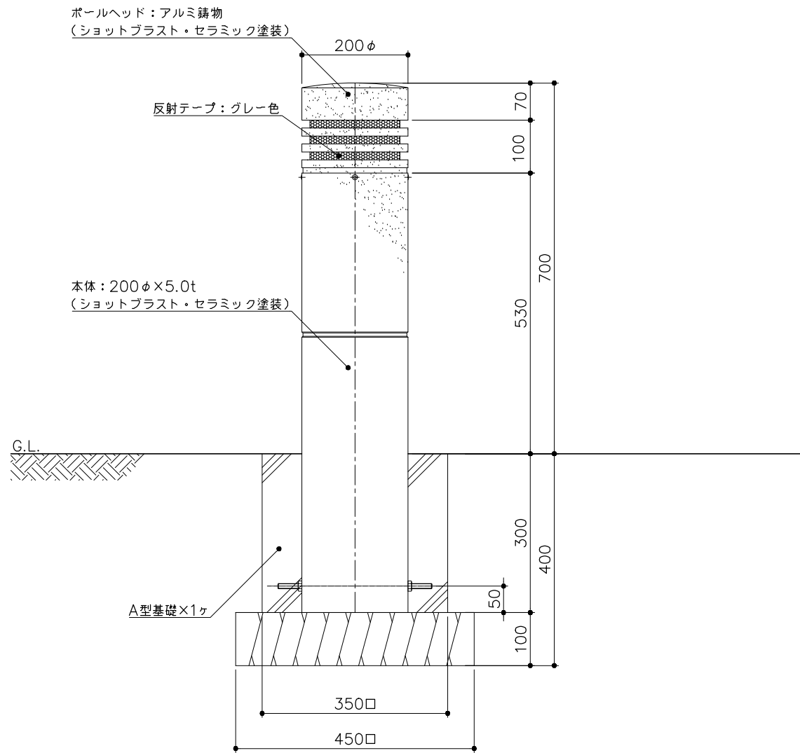
立面図 S= 1：10
