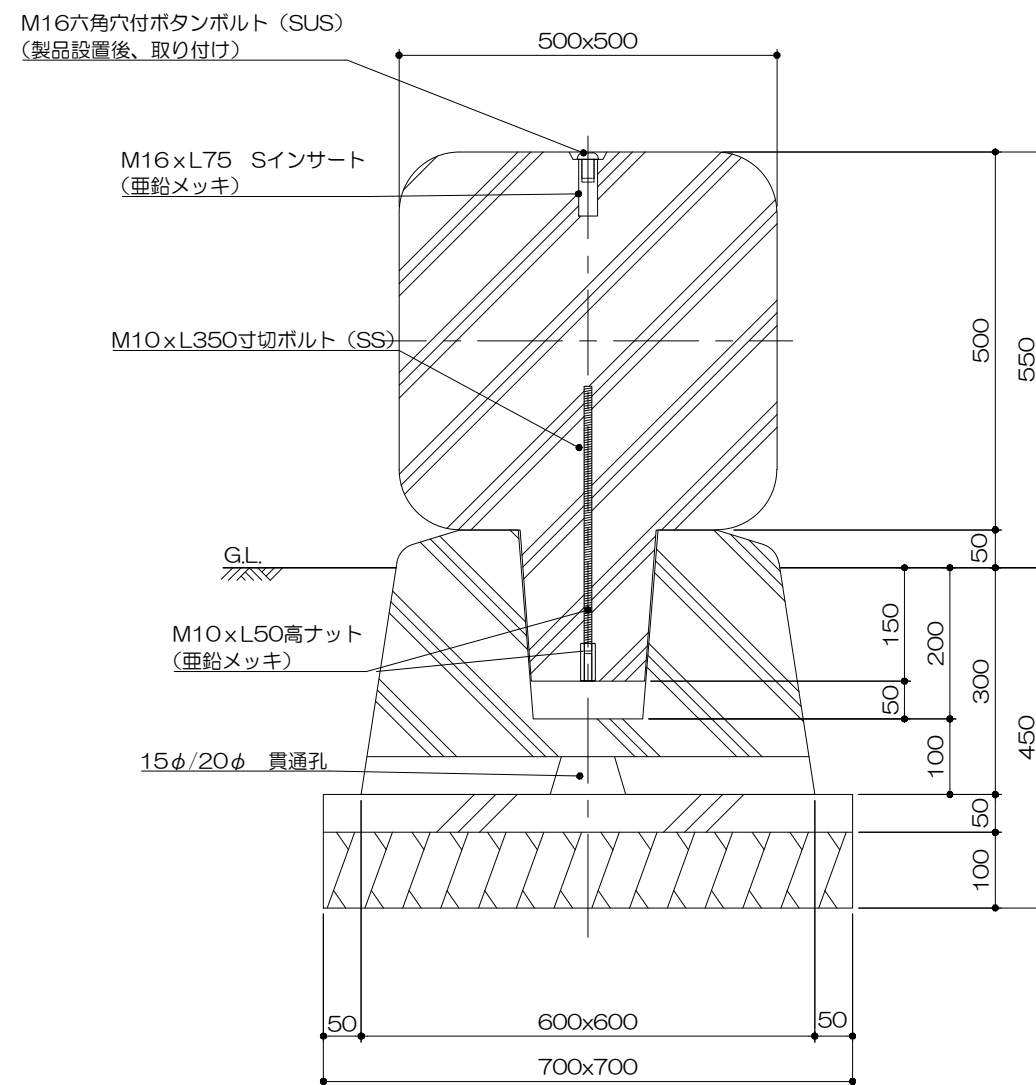
側面図 S= 1 : 10
