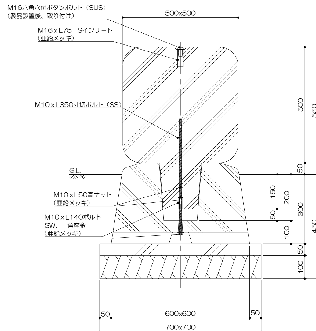
側面図
