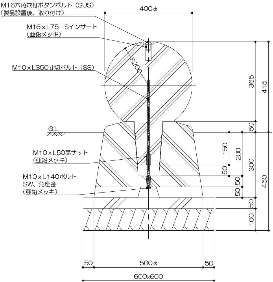
側面図 S= 1 : 10
