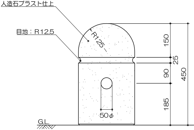
立面図 S= 1 : 10
