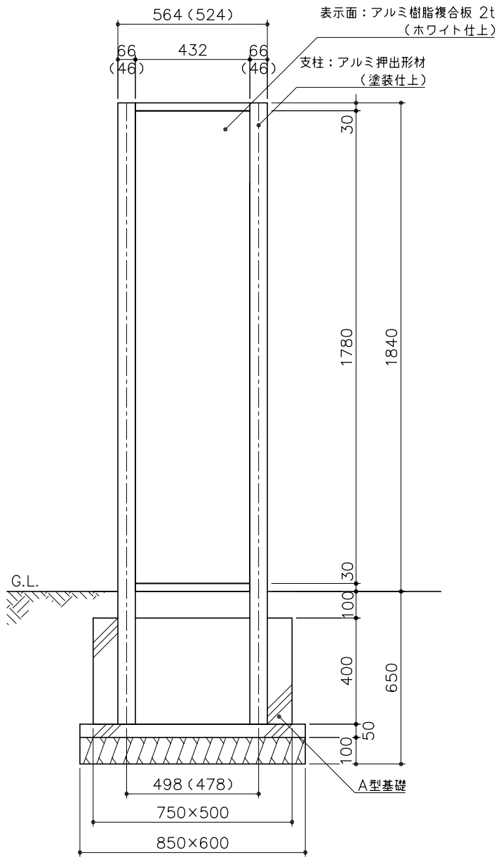
立面図 S= 1：20
