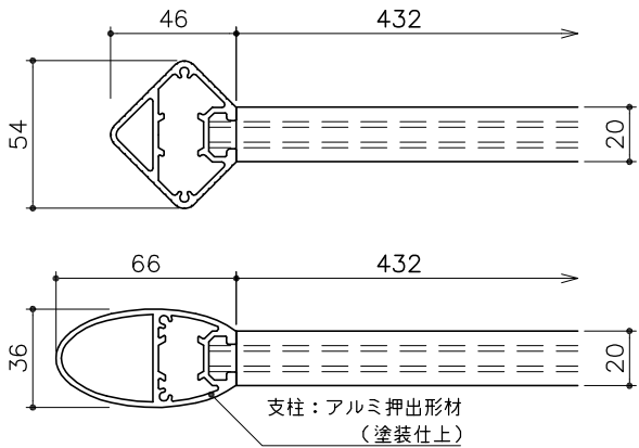
平面図 S= 1：3
