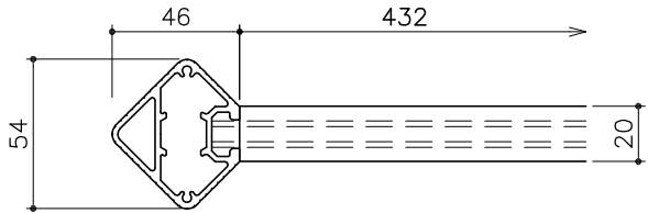
平面図 S= 1：3
